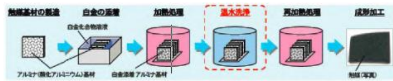
図(添付 1-1) 排ガス再結合器触媒の概略製造工程
