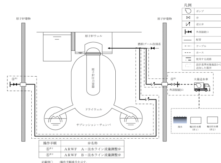
図 2.4-1 原子炉ウエル代替注水系の概要図
