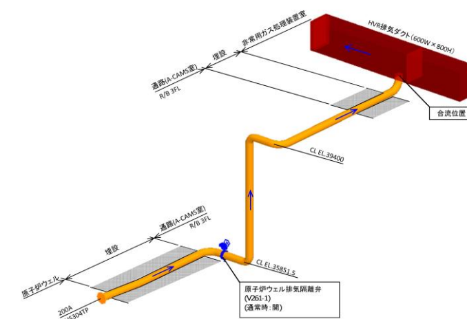
図 2 原子炉ウェル排気ラインのルート (アイソメ図)
