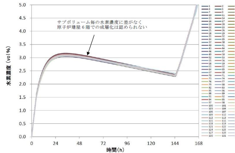
第 2.1.4.2-4 図 ケース 2 水素濃度の時間変化 (サブボリューム別)
