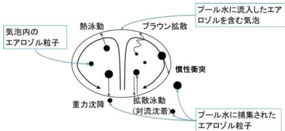
図3 スクラビング水中を浮上する気泡中のエアロゾル
