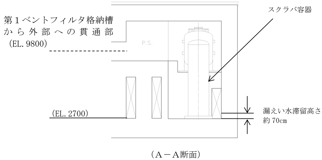
図4 第1ベントフィルタ格納槽から外部への貫通部と漏れい水の高さの関係
