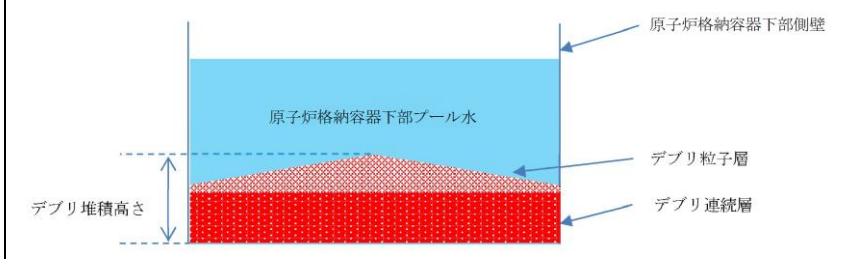
図 4 デブリ堆積高さの概念図 (不確かさ考慮)
