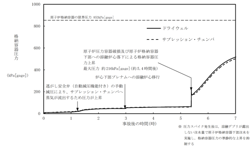
図 2 格納容器圧力の推移 (初期水張り水位約 3.8m)
