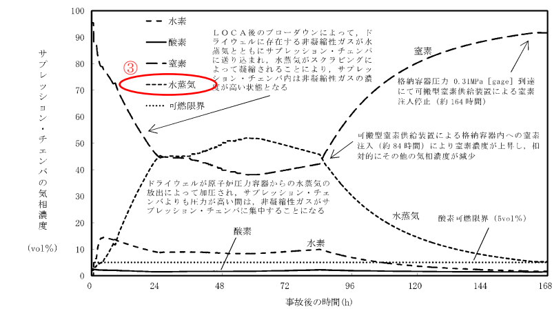
第 3.4-4 図 サプレッション・チェンバの気相濃度の推移 (ウェット条件)
