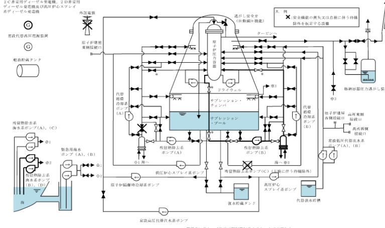
第5.1-1 図 崩壊熱除去機能喪失時の重大事故等対策の概略系統図 (2/2) (残留熱除去系 (原子炉停止時冷却) による原子炉除熱段階)
