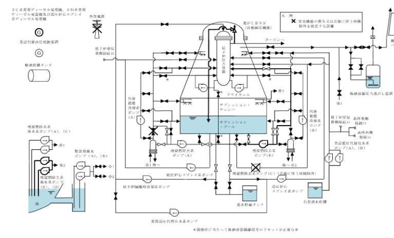
第5.1-1 図 崩壊熱除去機能喪失時の重大事故等対策の概略系統図 (1/2) (原子炉減圧及び残留熱除去系 (低压注水系) による原子炉注水段階)
