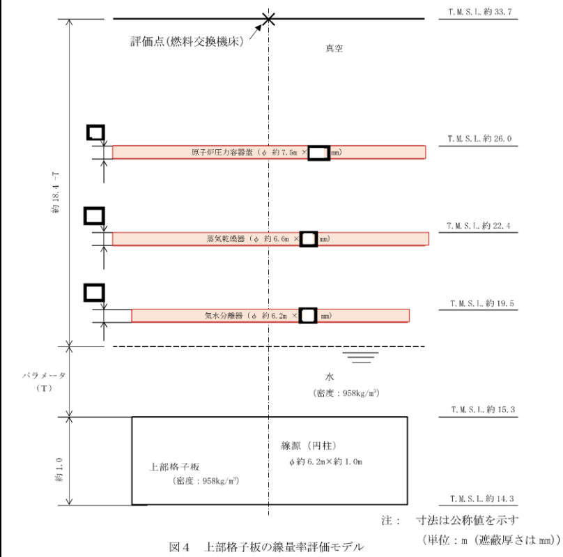
図4 上部格子板の線量率評価モデル
