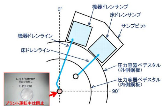
図 1-2 ドライウェルサンプの配置
