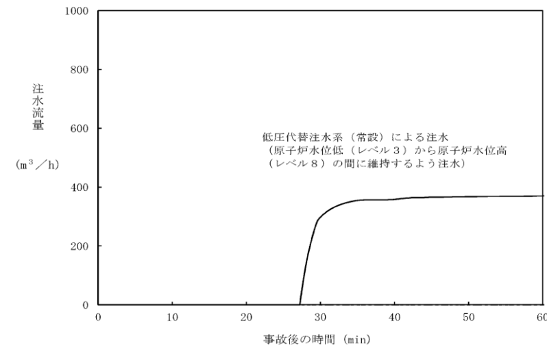
第 2.1-7 図 注水流量の推移
