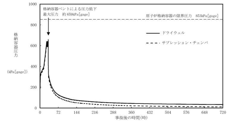
図 1.4 格納容器圧力の推移 (格納容器過圧・過温破損) (残留熱代替除去系を使用しない場合)
