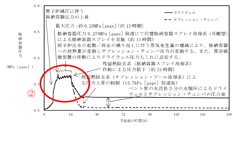
第 2.3.2-13 図 格納容器圧力の推移
