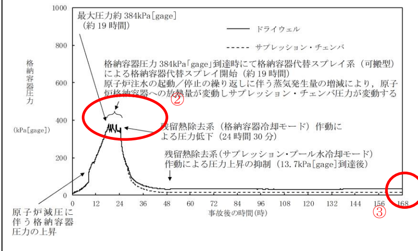
第 2.3.2.2-1(10) 図 格納容器圧力の推移
