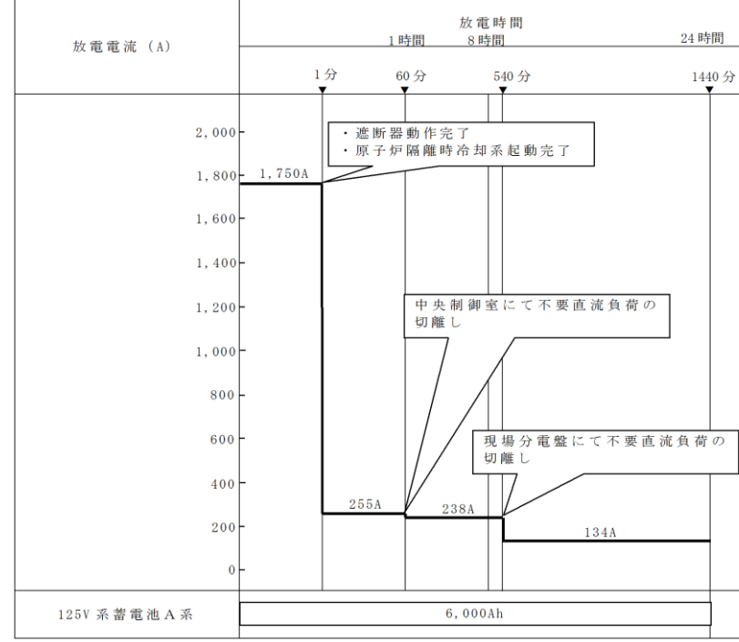
第 1 図 125V 系蓄電池 A 系 負荷曲線
