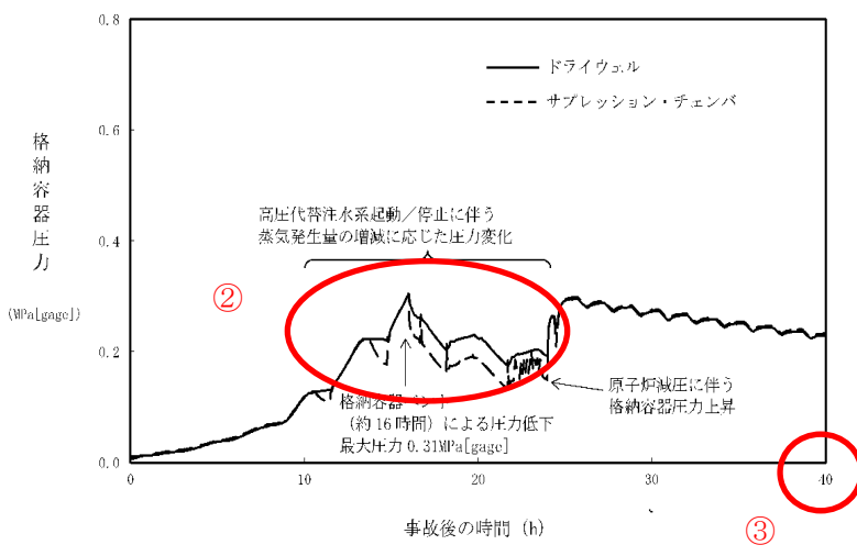
第 2.3.2.16 図 格納容器圧力の推移
