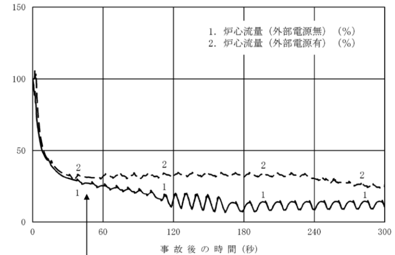
第 2.5.3-1(2) 図 外部電源がない場合の炉心流量の推移 (事象発生から 300 秒後まで)
