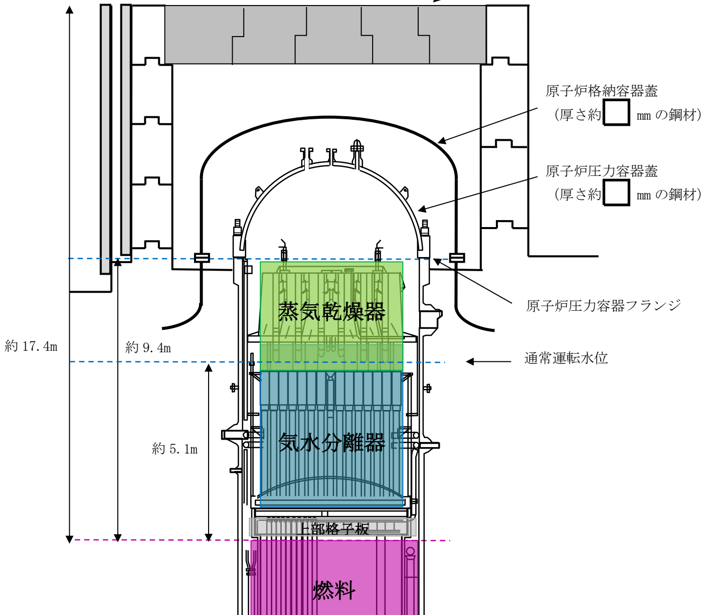
図2 原子炉圧力容器等構造物の概要
