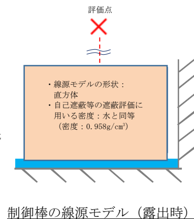
図5 使用済制御棒の冠水時及び露出時の線量率評価モデル
