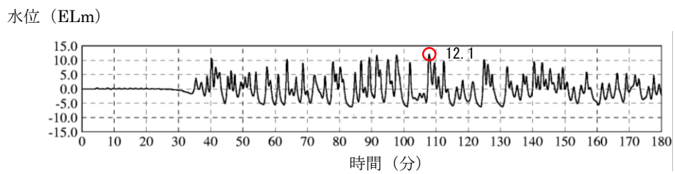
第6図 取水槽除じん機エリアでの時刻歴波形
