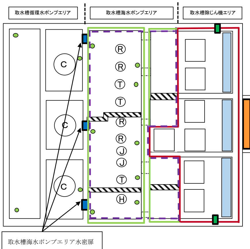
第 3 図 取水槽海水ポンプエリア水密扉配置図
