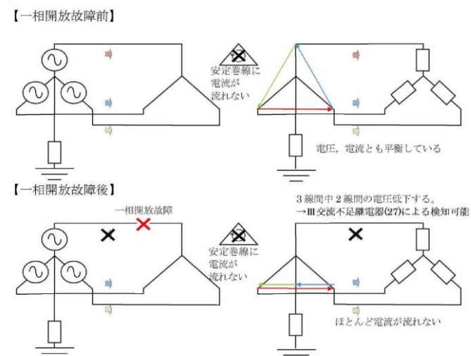
第2.2.1.1-11 図 交流不足継電器(27)による検知(イメージ) (予備変圧器)
