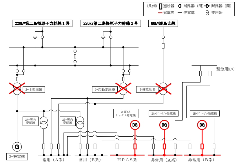
第2.2.4-4図 主変圧器、起動変圧器及び予備変圧器故障時の電力供給
