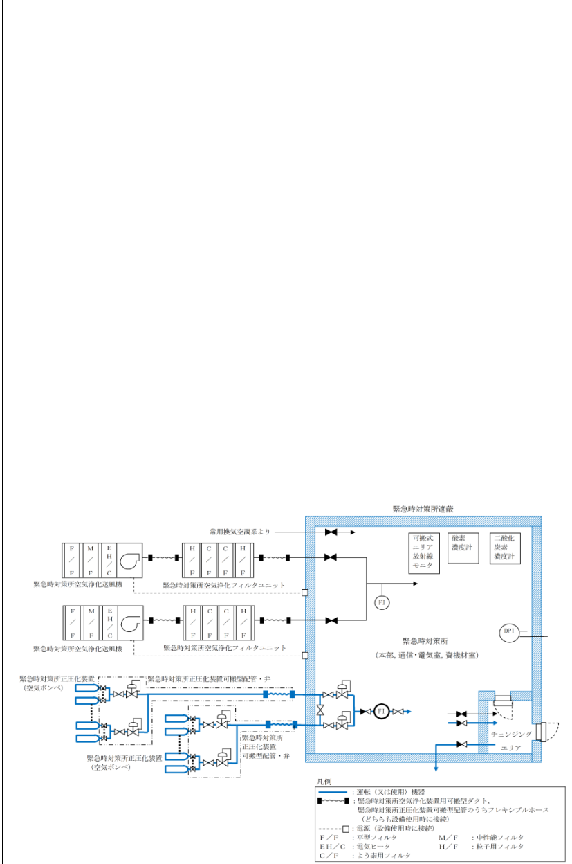
第2.4-2 図 緊急時対策所換気空調設備 系統概略図
