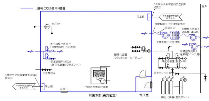
図2.4-2 5号炉原子炉建屋内緊急時対策所 (対策本部)
