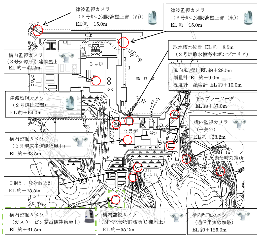
図 2.1-2 中央制御室から外の状況を把握する設備の配置図
