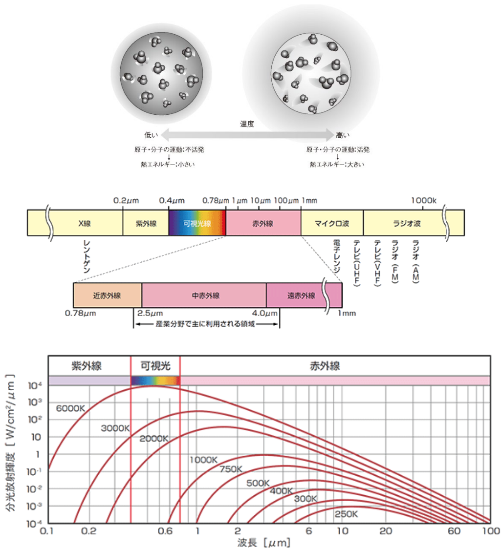
第 4 - 6 図 温度測定 の 原理
