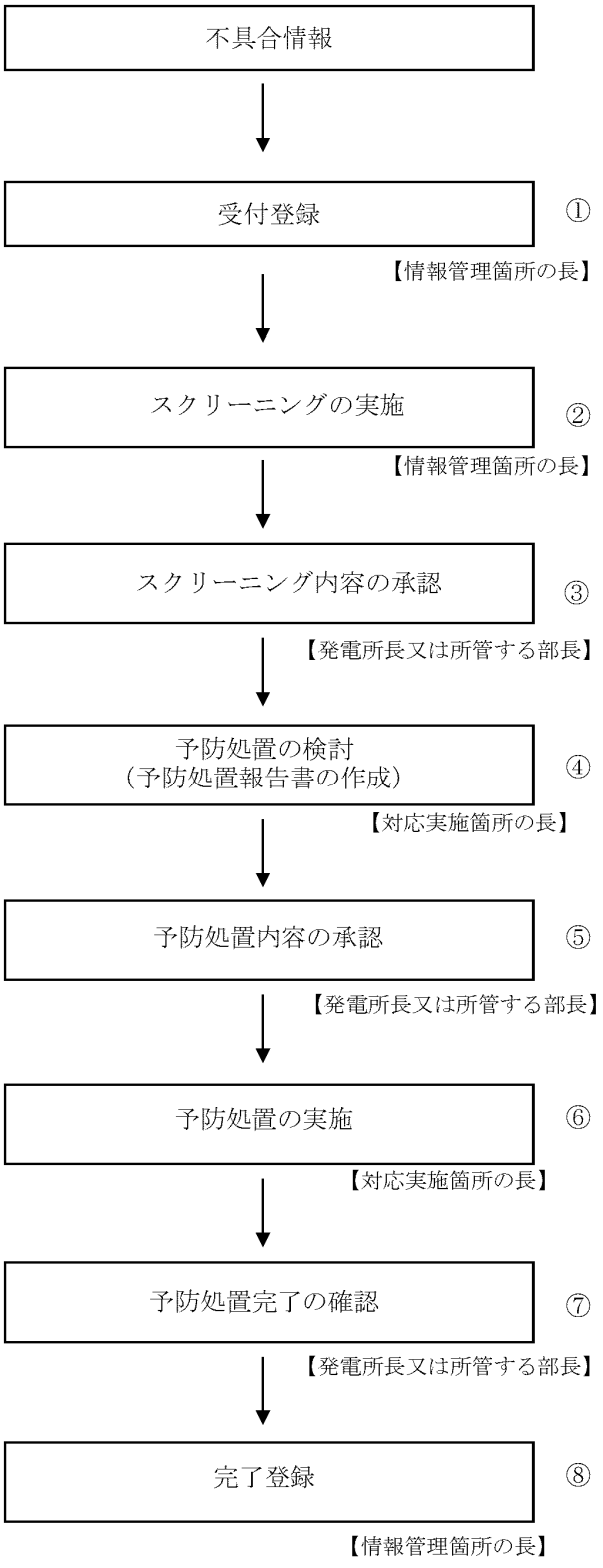
第6図 不具合情報の処理フロー
