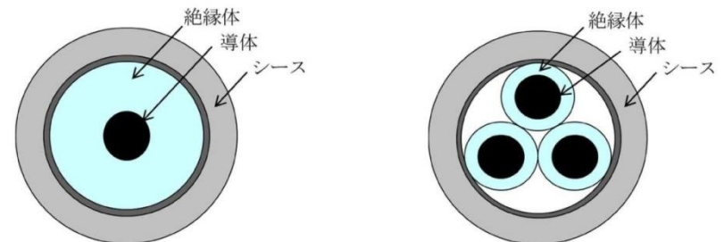
(a) 同軸ケーブル (b) 低圧ケーブル
