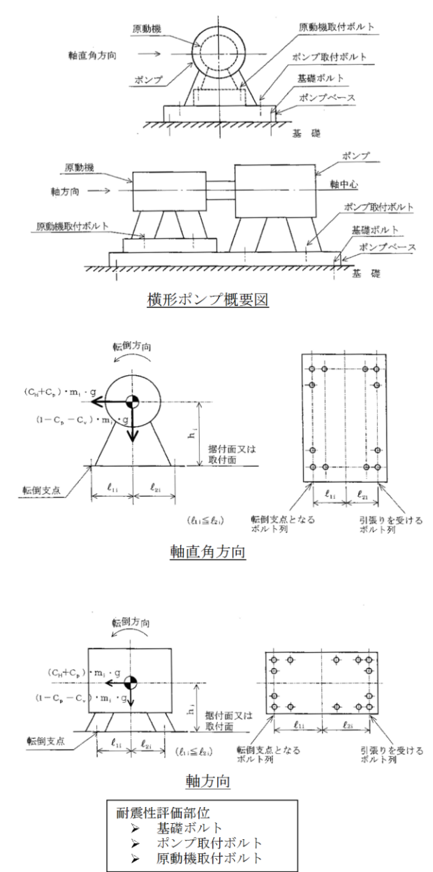
図 7-1 耐震評価の概要 (横型ポンプの例)
