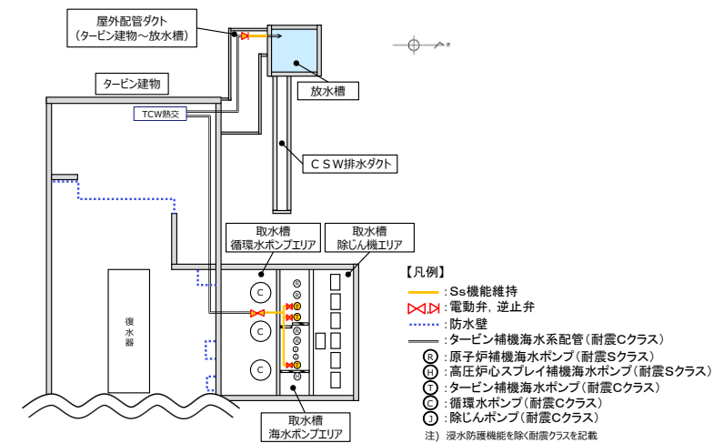
図 9-10-2 タービン補機海水系の対策概要 (平面図)
