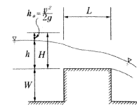
図 3-1.11 長方形せきの諸元
