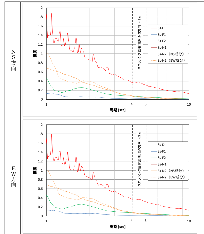
図 8-3 燃料プールの床応答スペクトル (減衰定数 0.5%*, EL 42.8m)
