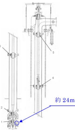
第4図 残留熱除去系海水系ポンプ 断面図
