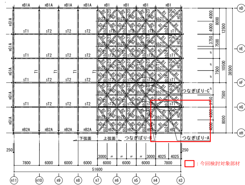
第 3-5 図 部材位置図 (トラス二次部材: 繫ぎ梁)
