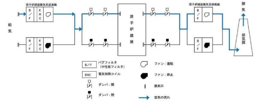
第2.4.2-3図 原子炉建屋換気系の系統概略図
