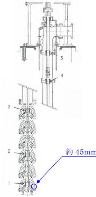
第4図 残留熱除去系海水系ポンプ 断面図
