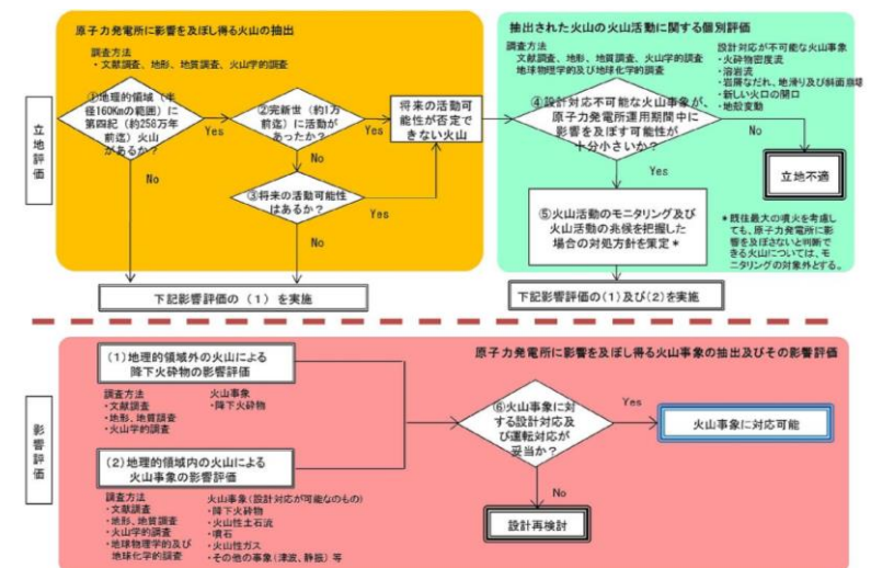
第 1.2-1 図 火山影響評価の基本フロー
