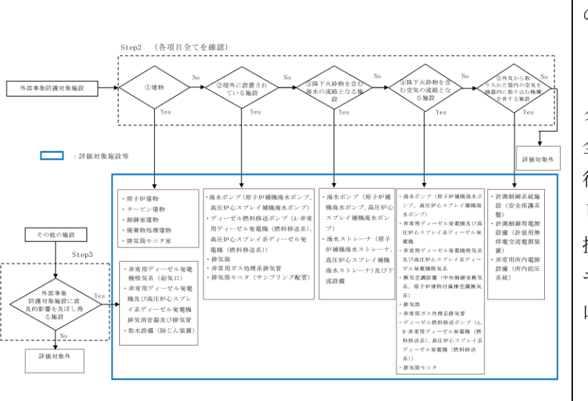
第 1.3-2 図 評価対象施設等の抽出フロー
