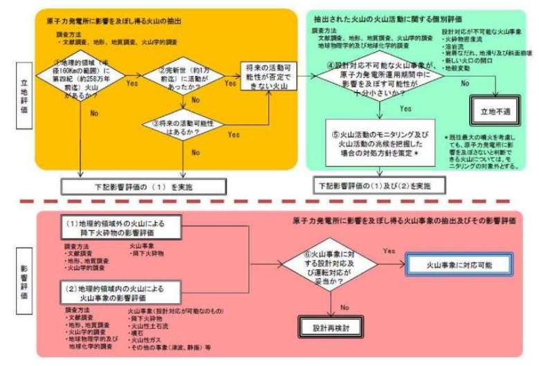
図 1.1 火山影響評価の基本フロー
