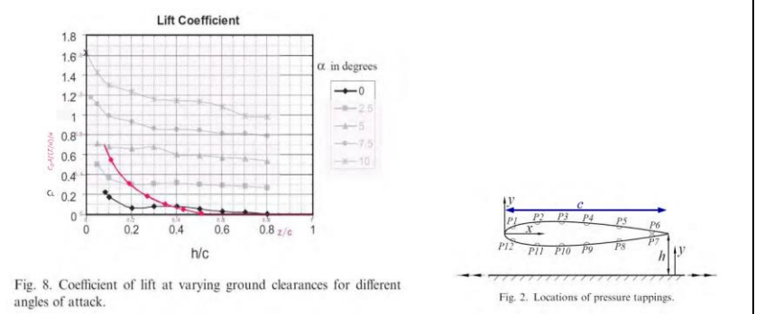
図19 翼の風洞試験による揚力係数と本モデルで代用した揚力係数の関係
