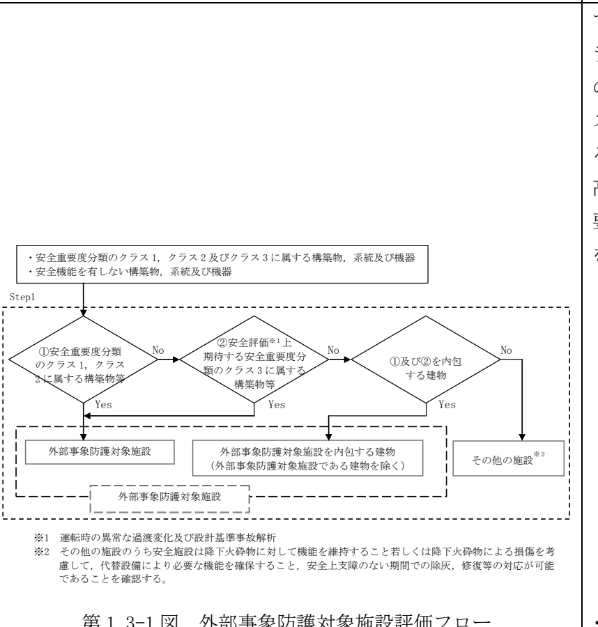
第 1.3-1 図 外部事象防護対象施設評価フロー
