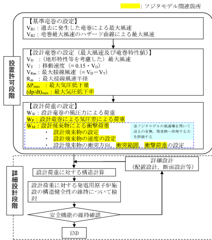
第2図 竜巻影響評価フローとフジタモデルの関連箇所
