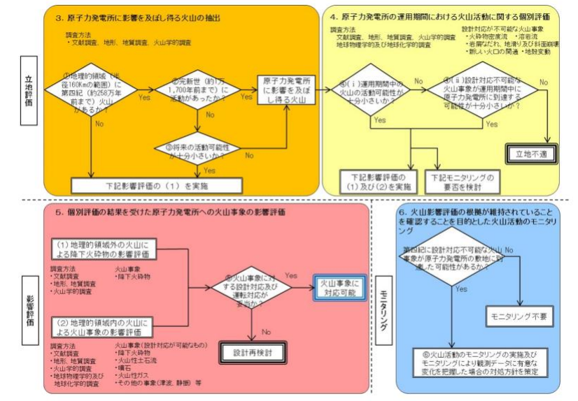
第 1.1 図 火山影響評価の基本フロー
