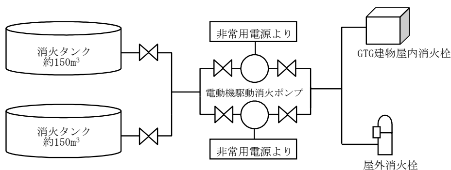
第6-2図 44m盤消火系の概要
