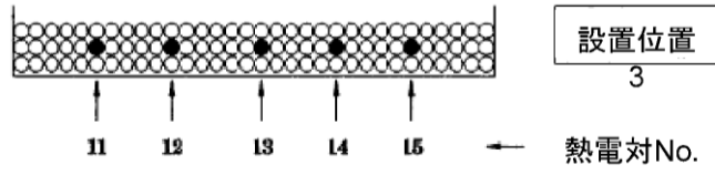
許容電流評価試験：ケーブルトレイ
