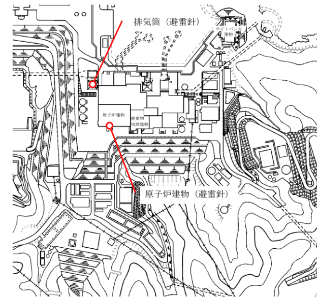
第 1-16 図 避雷設備の設置対象建物等
