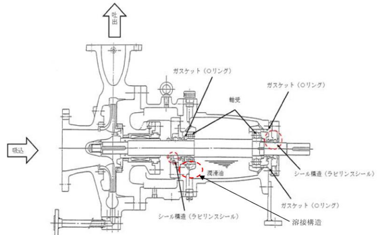
第1-1図 溶接構造、シール構造による漏えいの防止対策概要図
