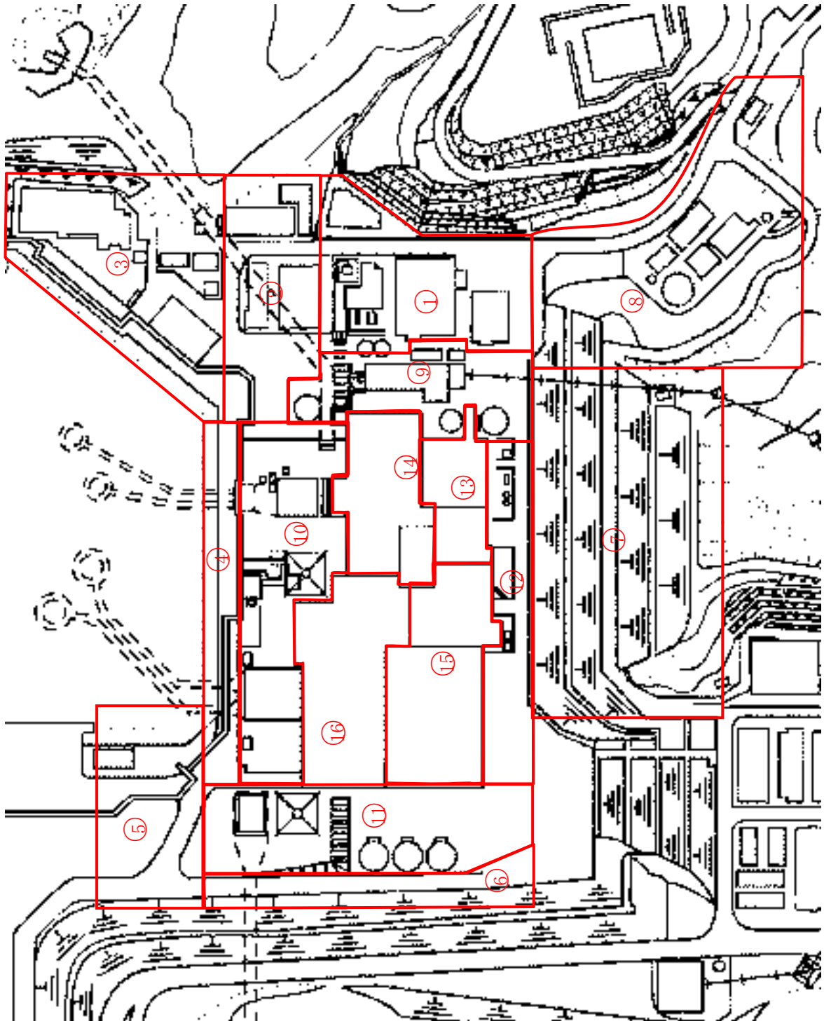
図 3.3.3 島根原子力発電所 竜巻飛来物発電所 竜巻飛来物現地調査区画図 (1, 2号炉周辺)
