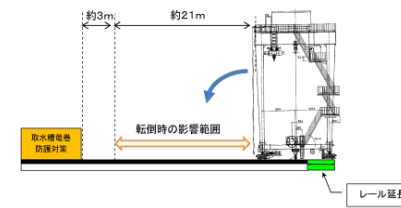
図6 ガントリークレーンの竜巻防護対策イメージ
