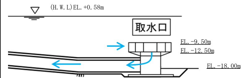
第2.5-2図 取水口断面図
