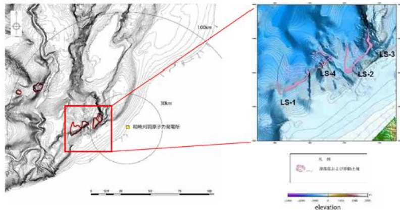
第2.5-8図 基準津波の波源
