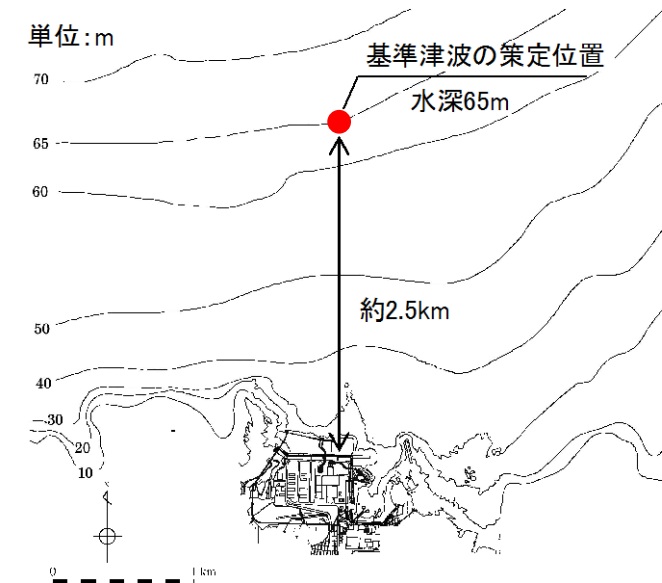
第2図 島根原子力発電所の基準津波策定位置
