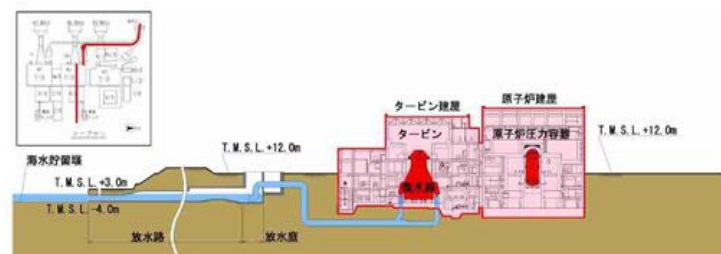
放水路断面
