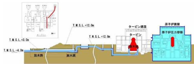
放水路断面
