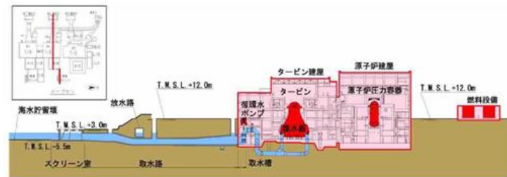
取水路断面
