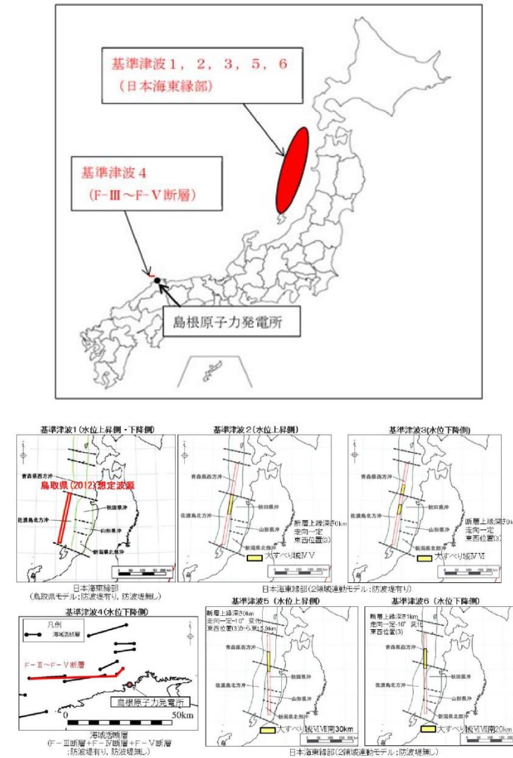
第3図 島根原子力発電所の基準津波の波源
