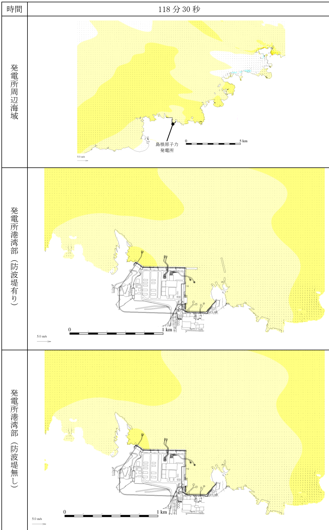
第 1 図 (38) 基準津波 1 の水位変動・流向ベクトル
