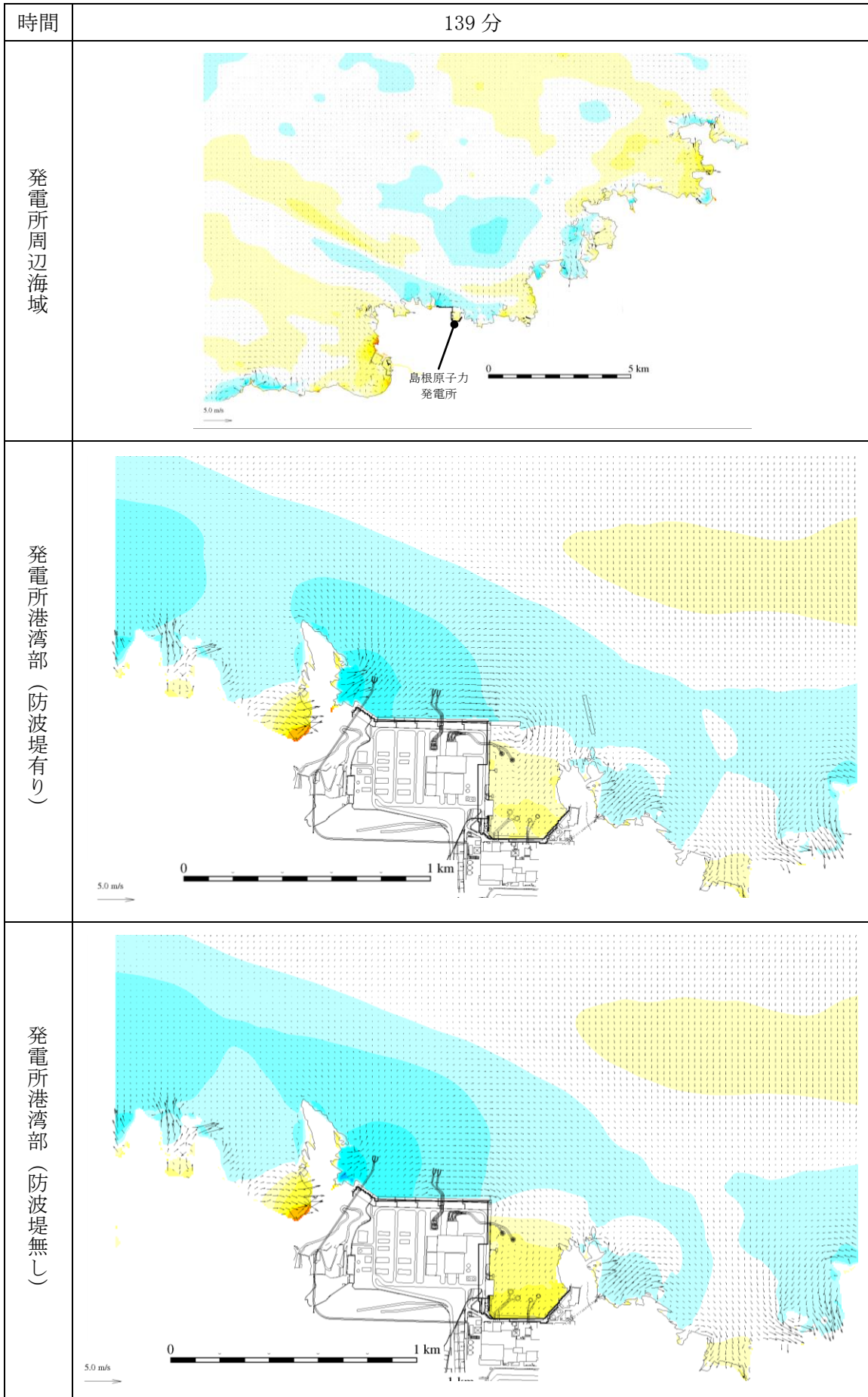
第 1 図(79) 基準津波 1 の水位変動・流向ベクトル
