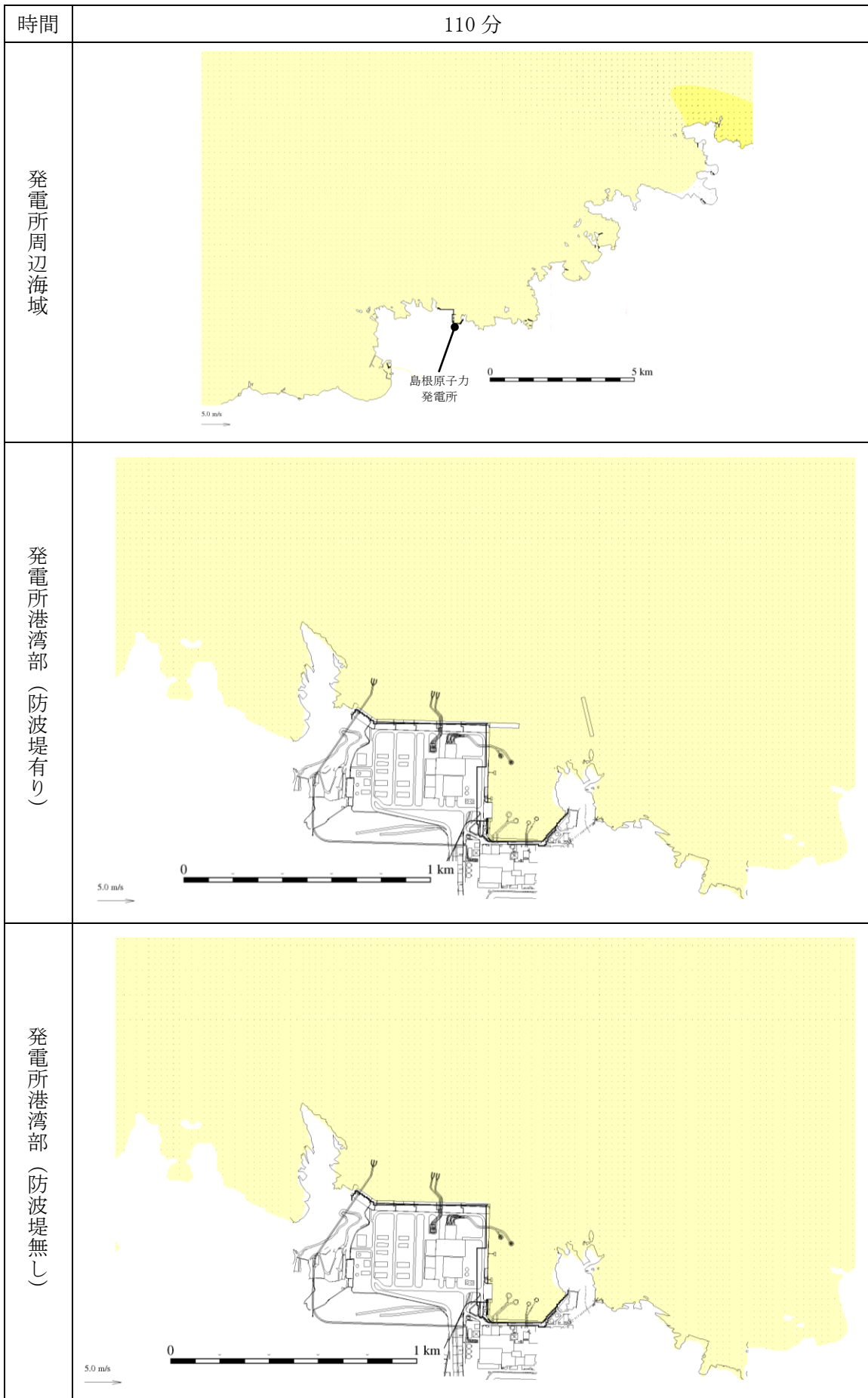
第 1 図(21) 基準津波 1 の水位変動・流向ベクトル
