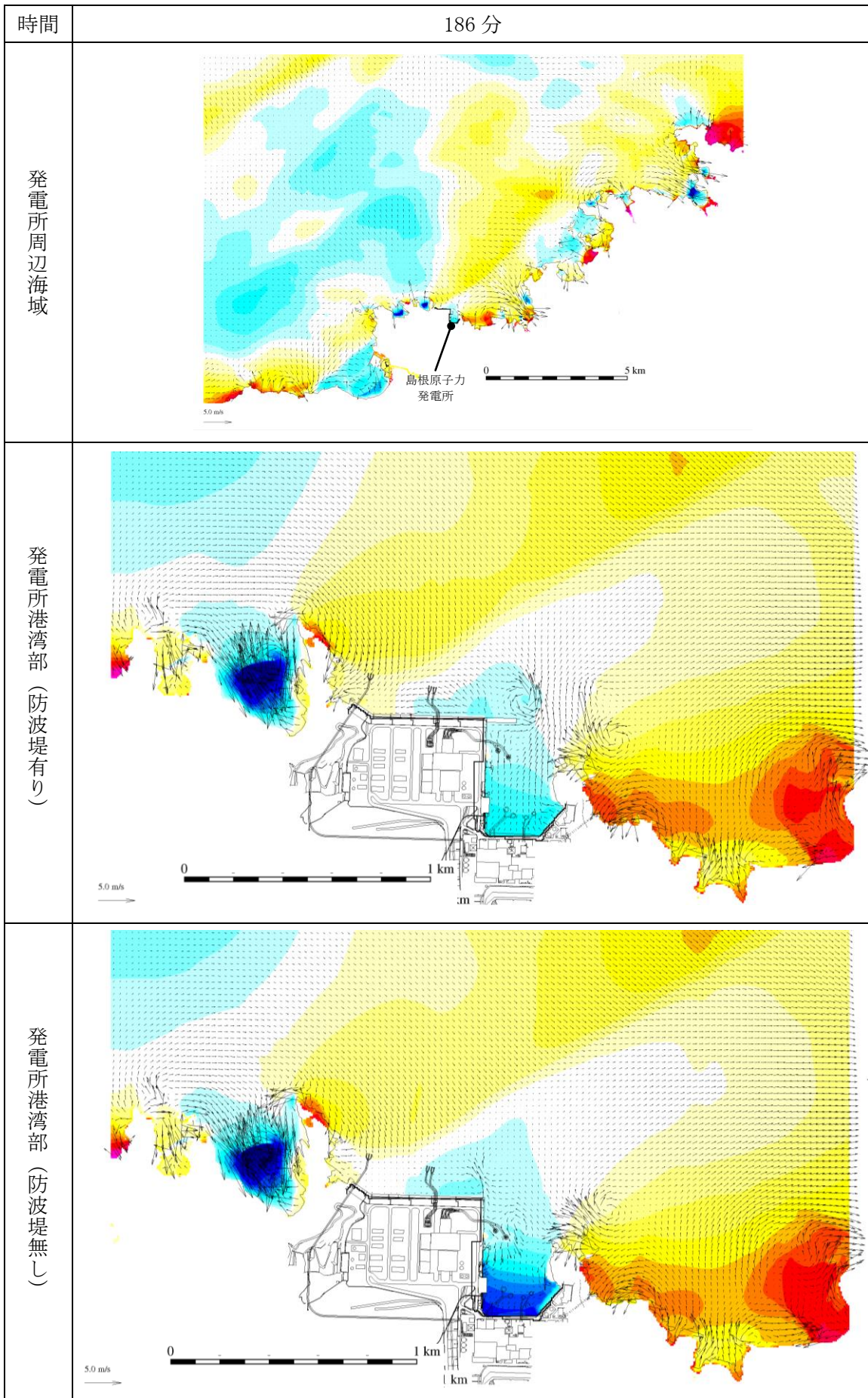
第 1 図 (173) 基準津波 1 の水位変動・流向ベクトル
