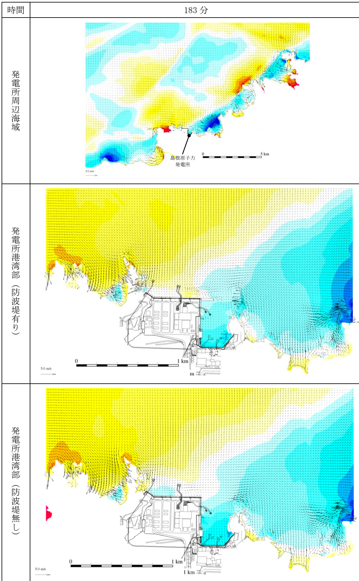
第 1 図(167) 基準津波 1 の水位変動・流向ベクトル
