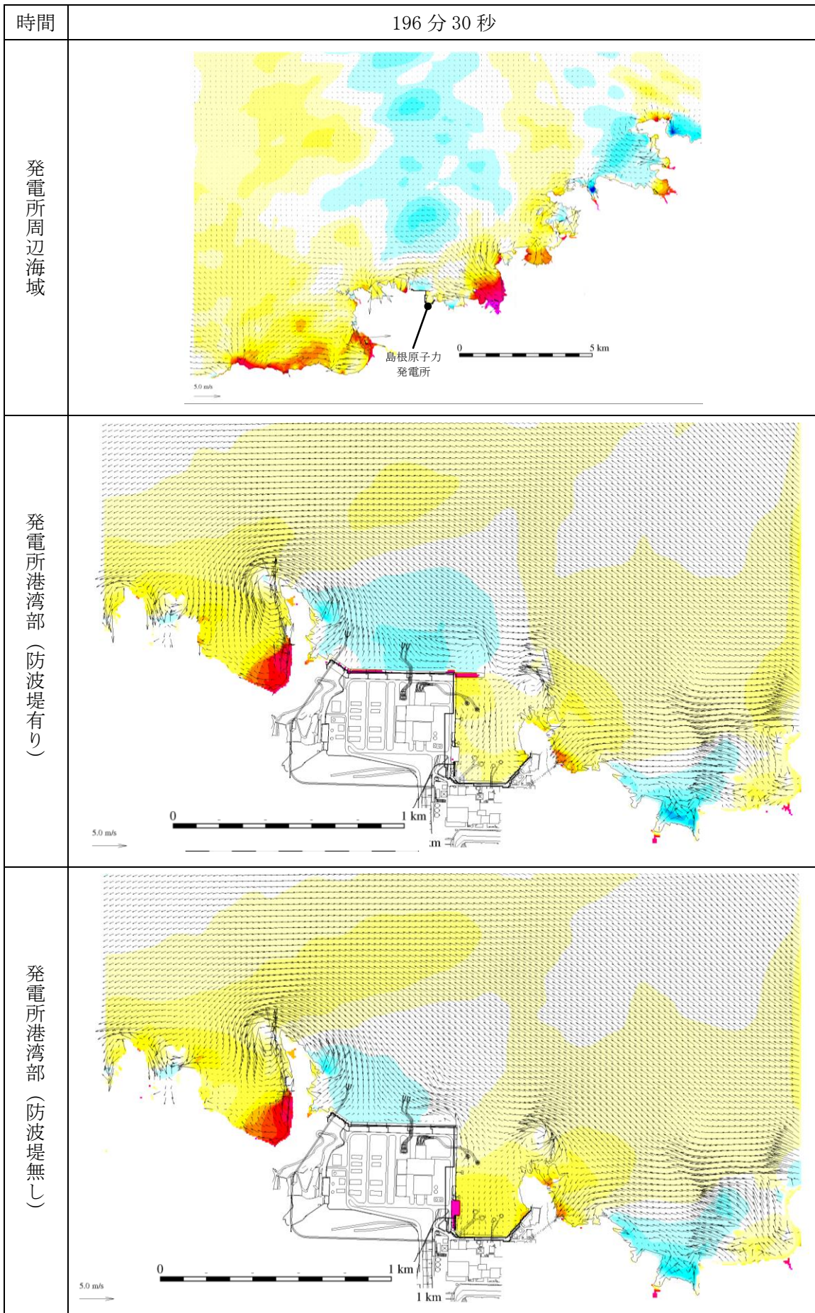
第 1 図(194) 基準津波 1 の水位変動・流向ベクトル
