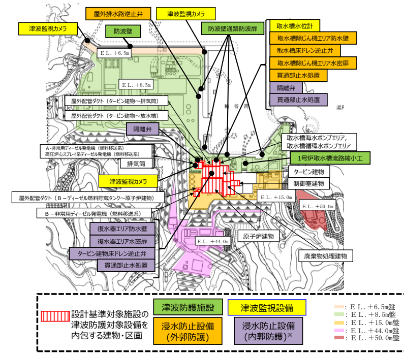
第3.4.1-1図 津波防護施設、浸水防止設備及び津波監視設備位置図
