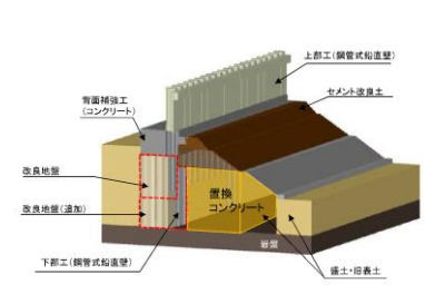
第3.4-3図 防潮堤（鋼管式鉛直壁）の上部工
