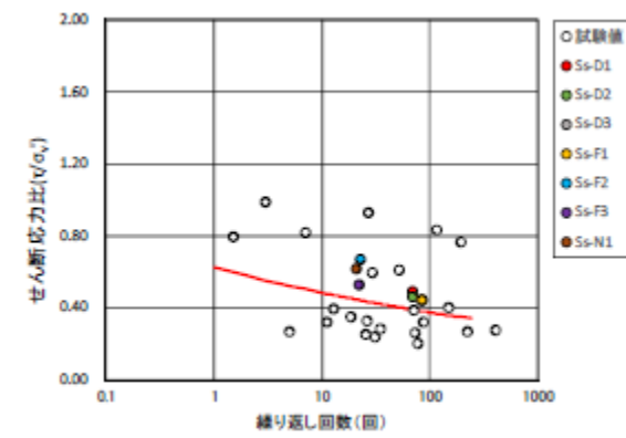
(b) 盛土
