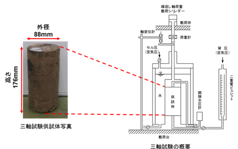
第3-2-3 図 繰返し非排水三軸試験の概要
