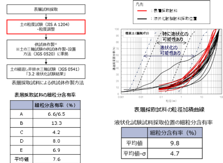
第3-1-6 図 表層採取試料と既往の試料採取位置の粒径加積曲線及び細粒分含有率
