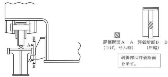
第4図 旧構造の評価に用いた評価断面図
