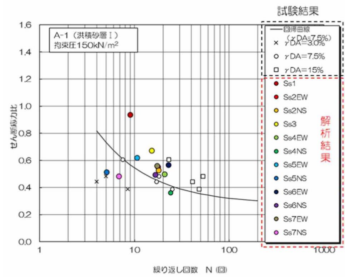
(b) 拘束圧150kN/m 2
