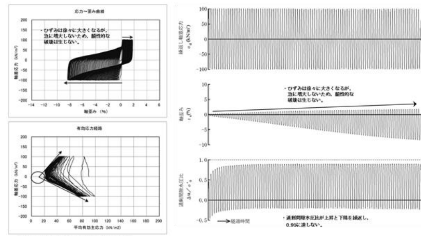
第3-2-9図 液状化試験結果の例 (E-4'地点の埋戻土 (掘削ズリ))
