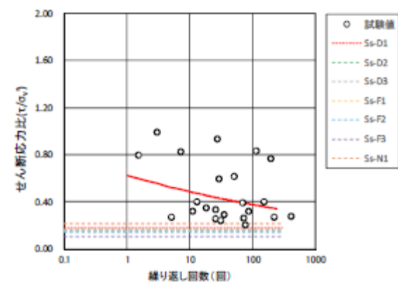
(b) 盛土
