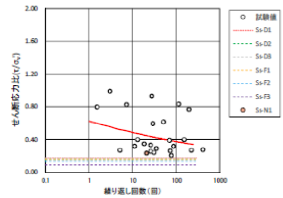
(a) 盛土
