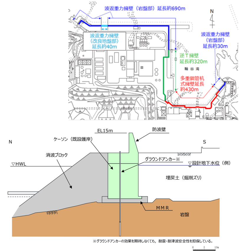
第4-2-12 図 防波壁 (波返重力擁壁 (岩盤部)) 断面図
