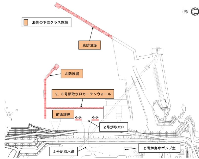
添付 6-2 図 海側の下位クラス施設配置図
