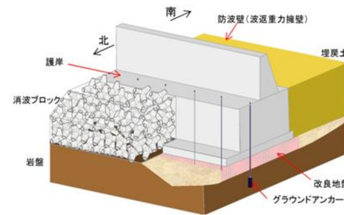
別紙 17-3 図 防波壁（波返重力擁壁）下部の地盤改良概要
