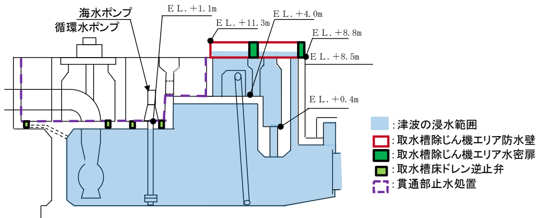
第 2.2-7 図 取水槽の流入防止の対策の概要 (断面図)
