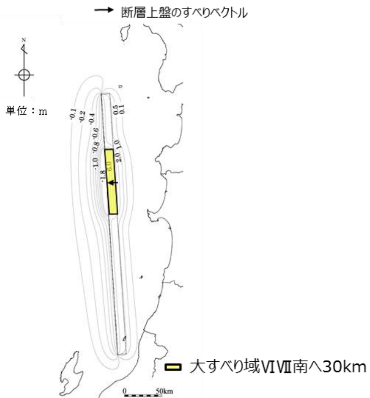
第 1.5-6 図 (6) 地殻変動量分布図：基準津波 5
