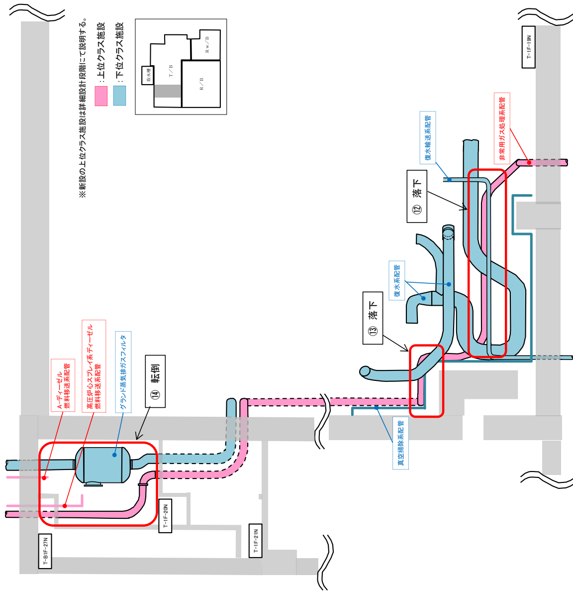
図 4-5 上位クラス施設と下位クラス施設的位置関係 (T/B 1FL 西側) (4/4)
