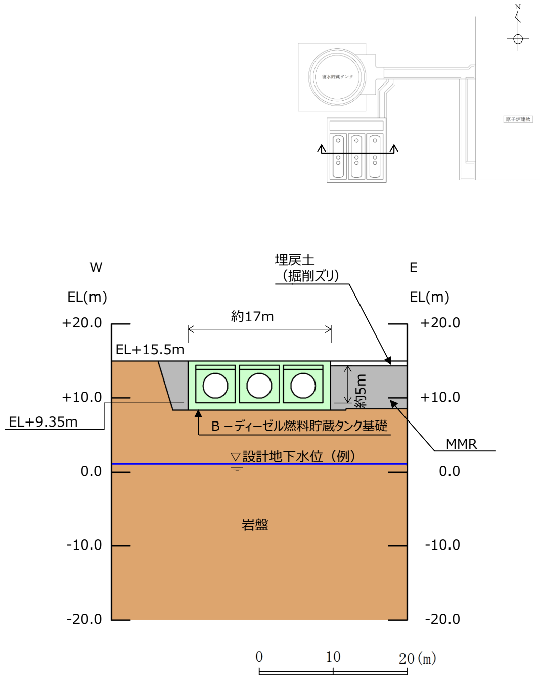
第4-2-7 図 B-ディーゼル燃料貯蔵タンク基礎 断面図
