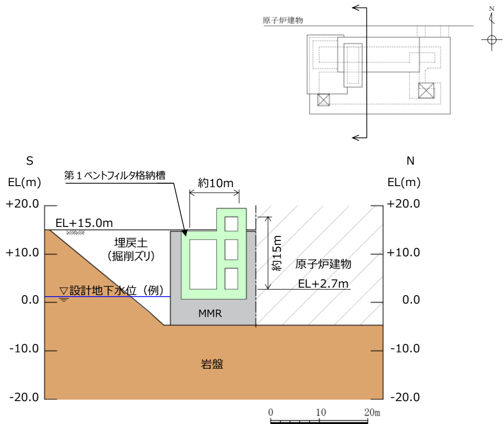
第4-2-15 図 第1 ベントフィルタ格納槽 断面図
