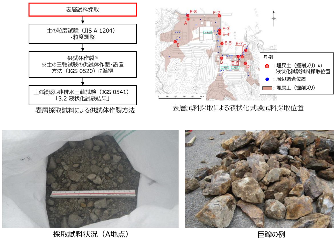
第 3-1-5 図 採取状況及び巨礫の例
