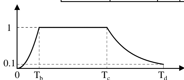
第 2-1 図 弾性設計用地震動 S d - 1 の模擬地震波の振幅包絡線の経時変化
