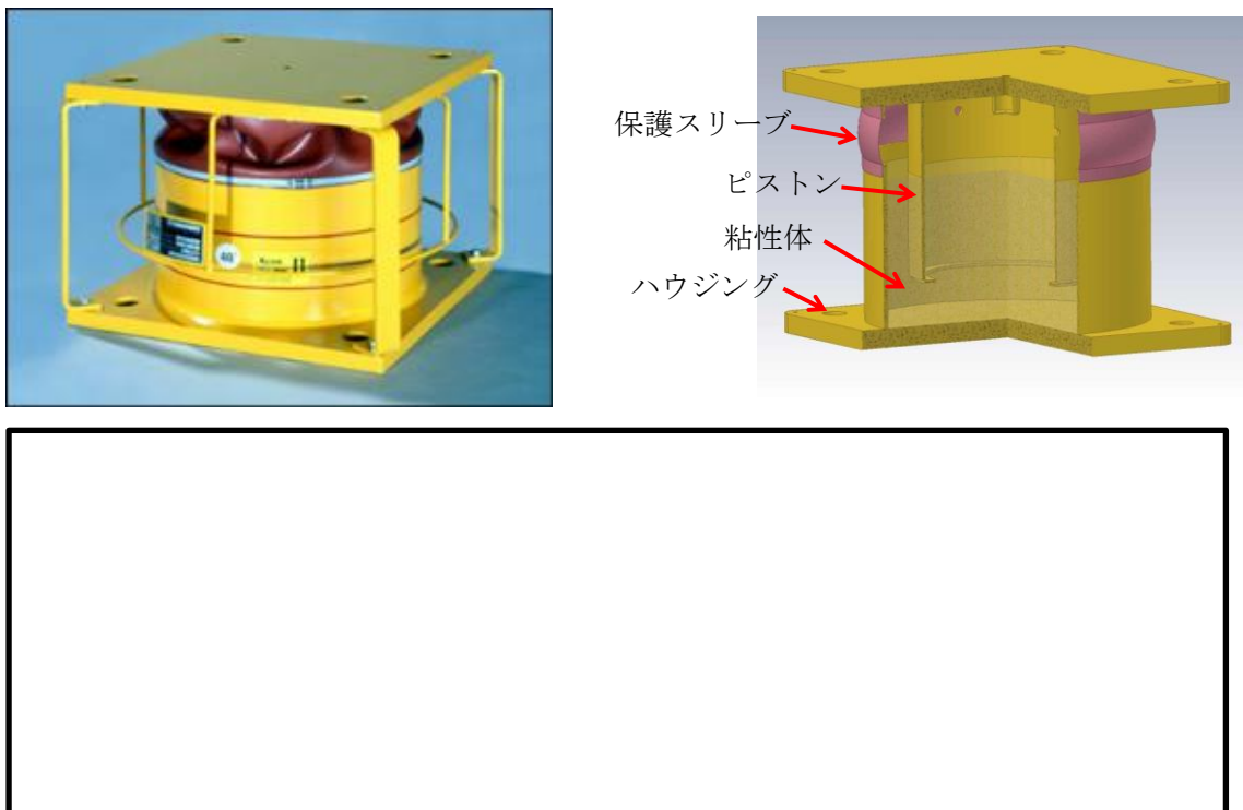
第3-3図 三軸粘性ダンパの外観及び構造
