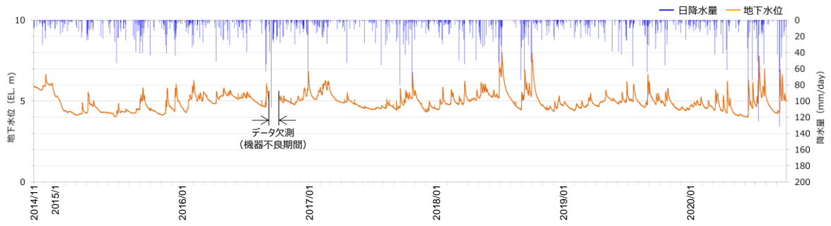
補足 9-2(7)図 地下水位観測記録 (No. 7 孔)
