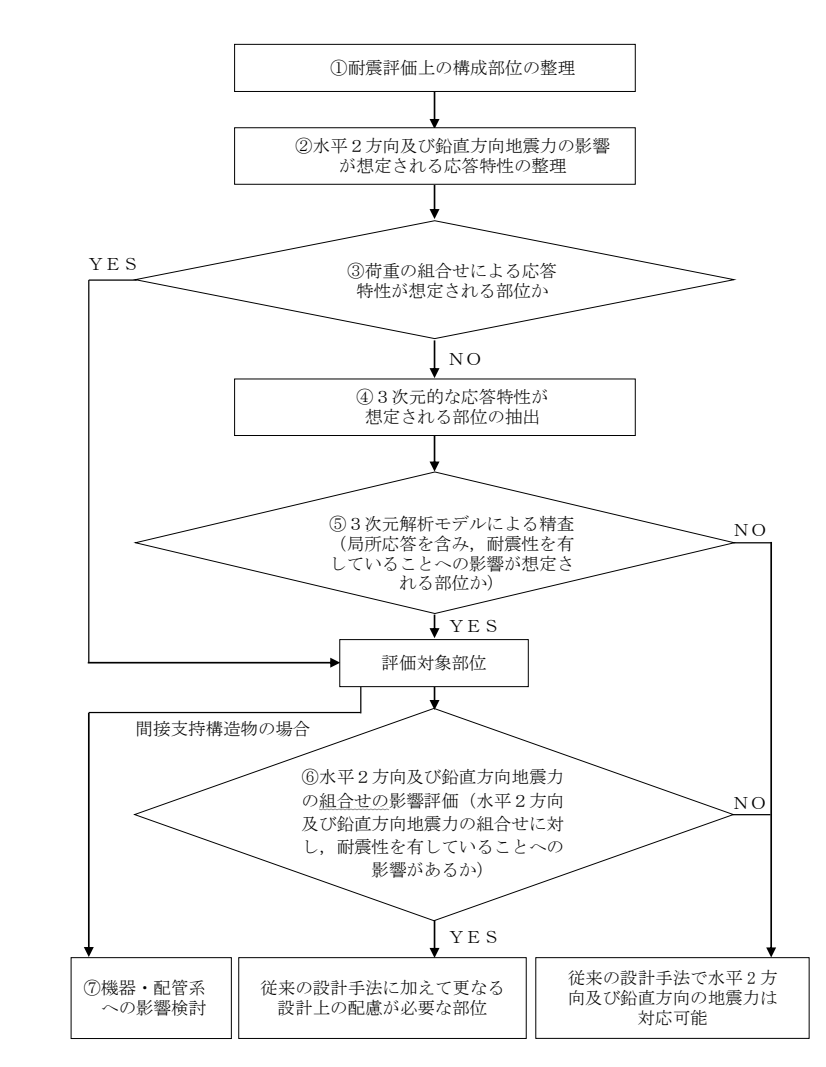
第4-2図 水平2方向及び鉛直方向地震力の組合せによる影響評価のフロー
