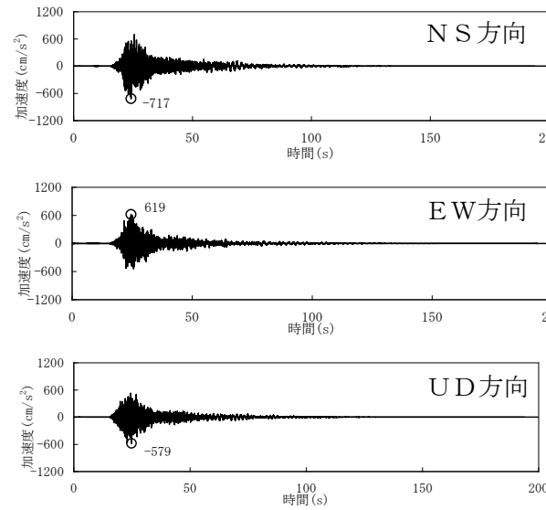
第5図 断層モデルを用いた手法による基準地震動 Ss の時刻歴波形 (Ss-11)
