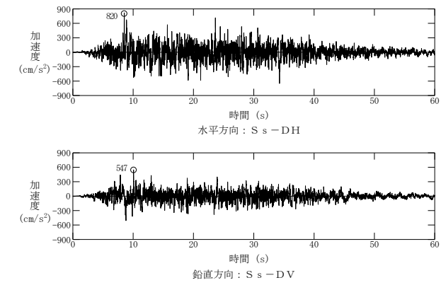
第3図 基準地震動 Ss-D の設計用模擬地震波の加速度時刻歴波形
