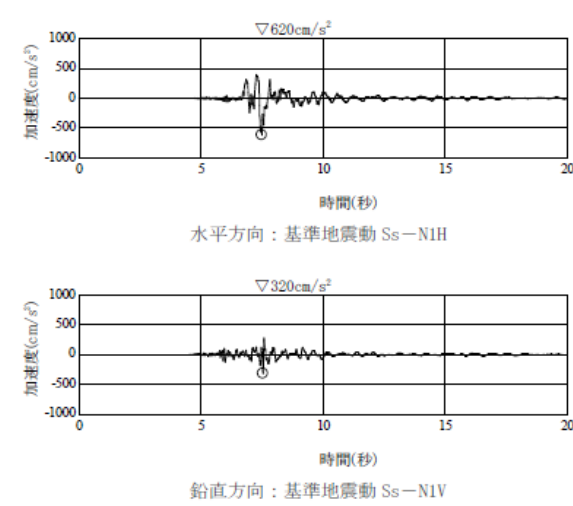
第5図 震源を特定せず策定する地震動による基準地震動 S_s の加速度時刻歴波形 ( S_s-N1 )
