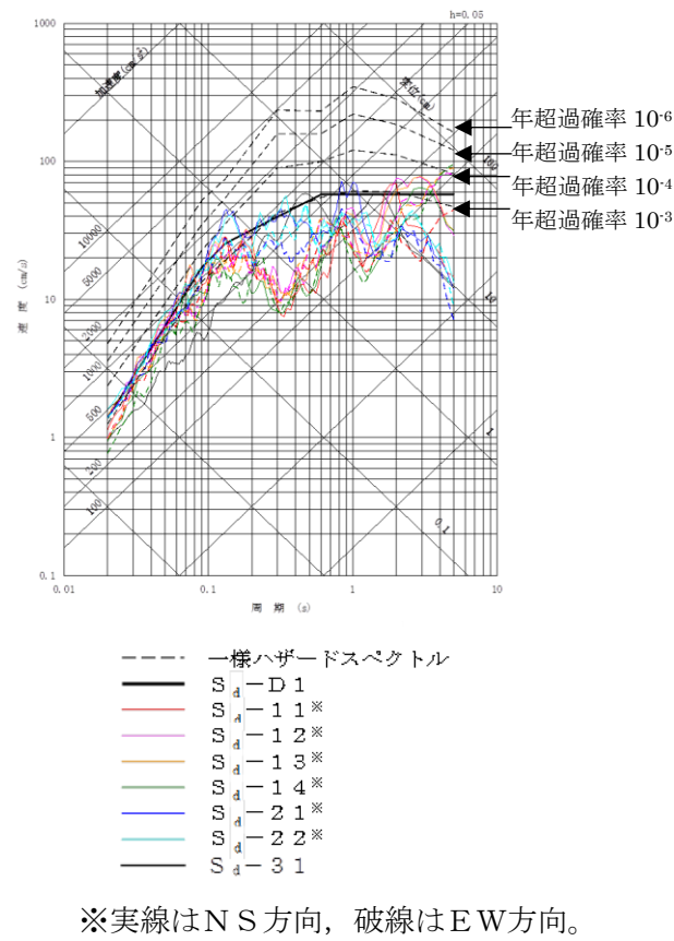
第1.3-14図 一様ハザードスペクトルと弾性設計用地震動S d の応答スペクトルの比較(水平方向)
