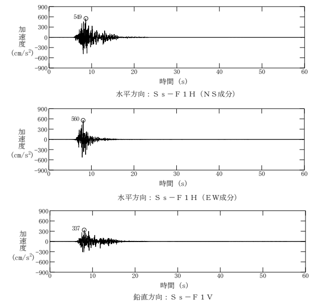
第4図 基準地震動 Ss-F1 の加速度時刻歴波形
