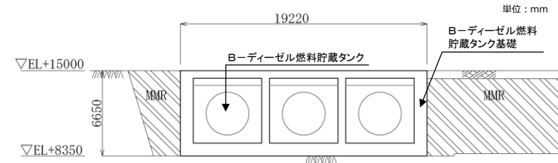
第6-2-24図 B-ディーゼル燃料貯蔵タンク基礎 断面図 (②-②断面)
