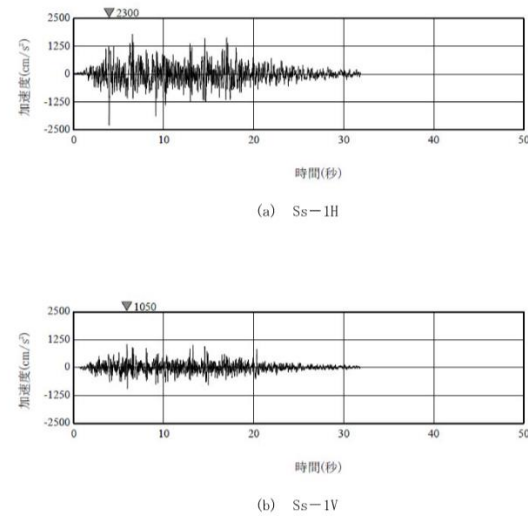
第4図 基準地震動 Ss-1 の加速度時刻歴波形 (荒浜側)
