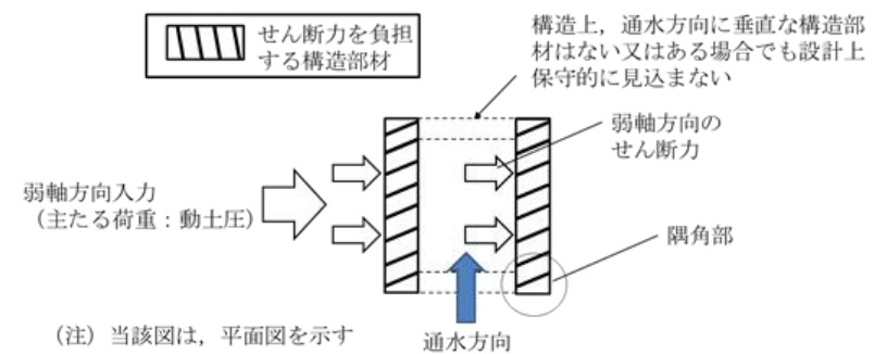
第4-5図 従来設計手法の考え方
