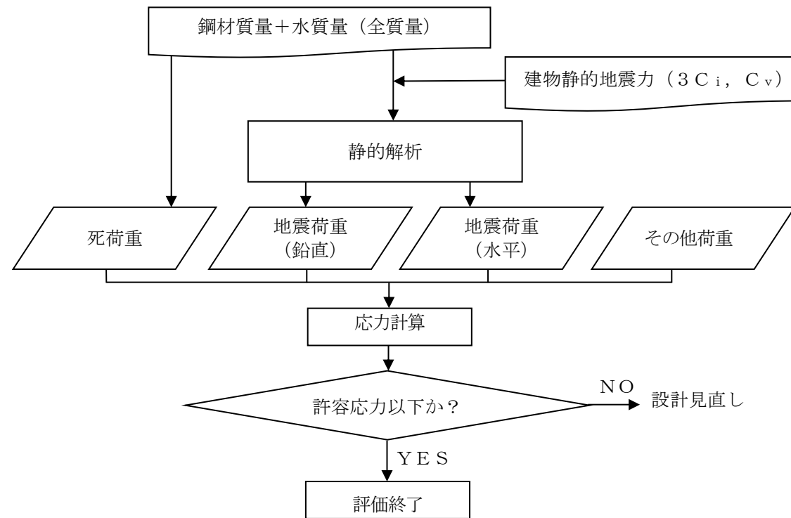
第 2.3-4 図 今回工認におけるサプレッションチェンバの静的地震力による耐震評価フロー(既工認と変更なし)
