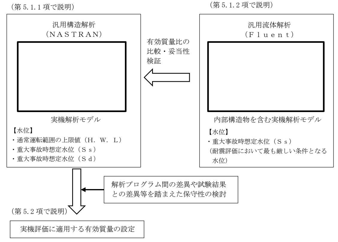
第 3.1-1 図 NASTRAN によるサプレッションチェンバ内部水の有効質量算出の妥当性検証及び島根 2号炉のサプレッションチェンバの耐震評価に用いる有効質量の設定の流れ
