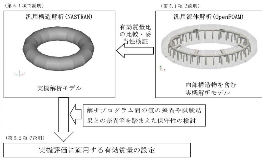
第 3.1-1 図 NASTRAN によるサプレッションチェンバ内部水の有効質量算出の妥当性検証及び女川 2号炉のサプレッションチェンバの耐震評価に用いる有効質量の設定の流れ
