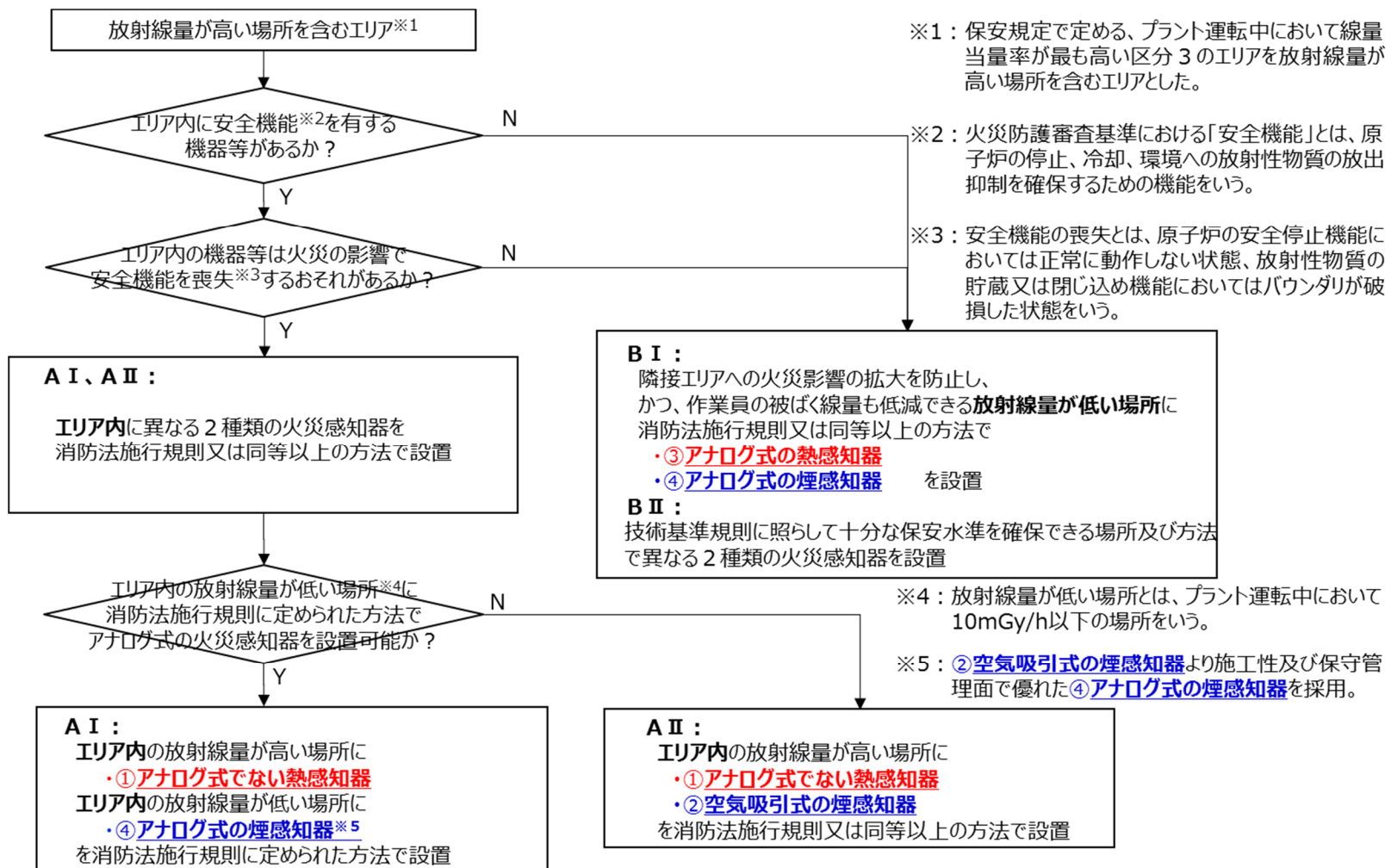
第 5-1 図 放射線量が高い場所を含むエリアの火災感知器設計フロー
