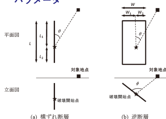
図4 破壊伝播補正モデルに用いるパラメータ 15)
