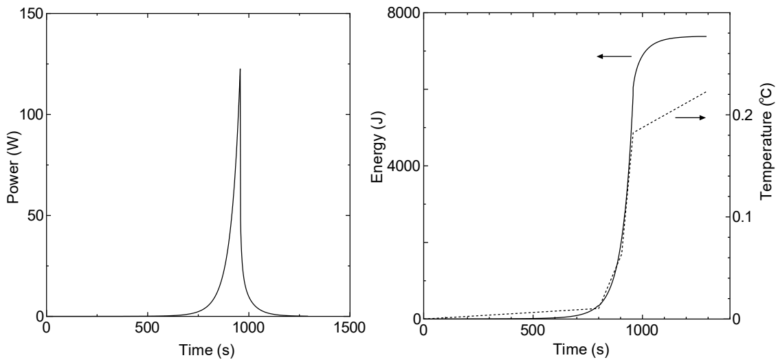
図 2-3-4 C45G(2H 2 O) 4 列炉心 出力変化 実験物の異常等による反応度の付加（ケース B ランプ状反応度添加） 出力変化（左）、積算出力と温度変化（右実線：出力、右点線：温度）
