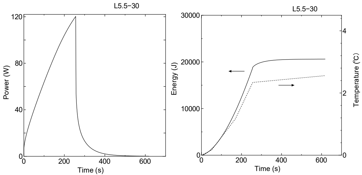
図 2-5-7 L5.5P-30 炉心 (ケース A \times 0.071 倍) 誤差考慮 (温度係数を 32% 減少) 出力変化 (左)、積算出力と温度変化 (右実線 : 出力、右点線 : 温度)
