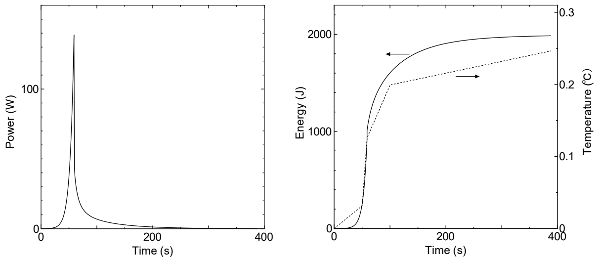
図 2-3-1 L5.5P-30 炉心
