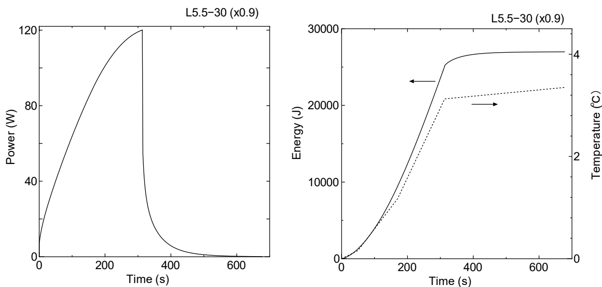
図 5-5 L5.5P-30 炉心 (中性子発生量 ケース A の×0.9 倍) 出力変化 (左)、積算出力と温度変化 (右実線 : 出力、右点線 : 温度)
