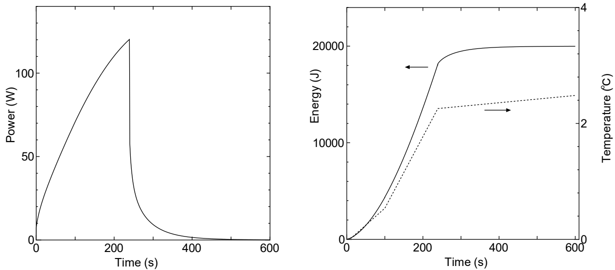
図 5-1 L5.5P-30 炉心
