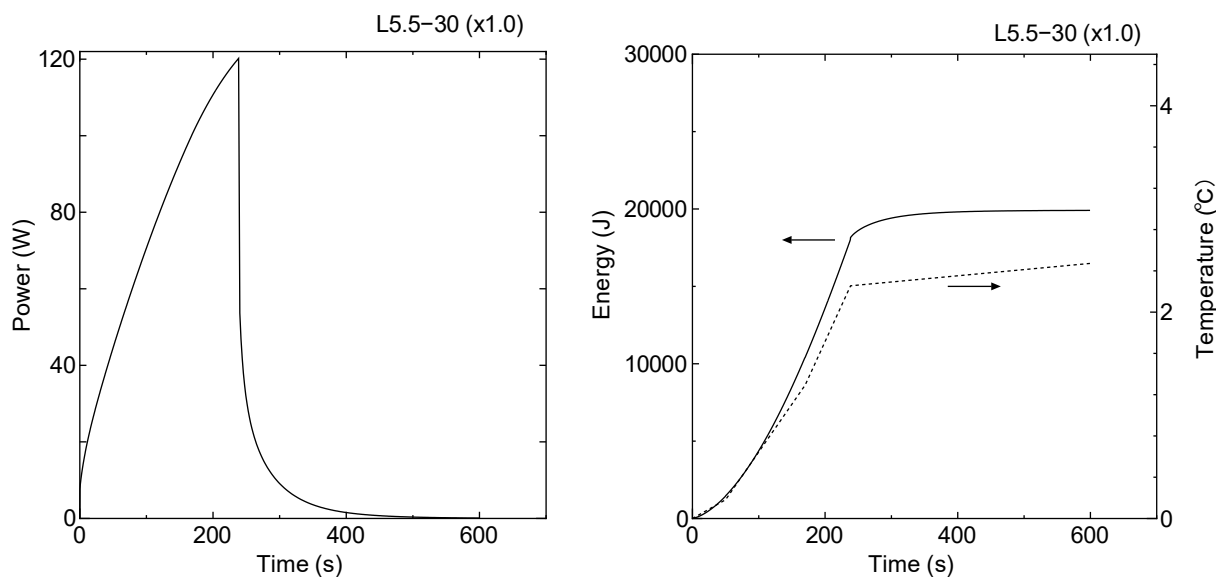
図 5-6 L5.5P-30 炉心 (中性子発生量 ケース A の×1.0 倍) (図 5-1 と同じ) 出力変化 (左)、積算出力と温度変化 (右実線 : 出力、右点線 : 温度)
