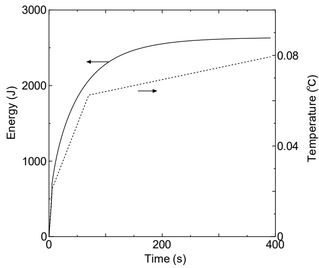
図 2-2 C45G(2H 2 O) 4 列炉心 出力変化（上、スケールの違う 2 つの図）、 積算出力と温度変化（下、右実線：出力、右点線：温度） （右図の横軸は制御棒挿入時からの経過時間）
