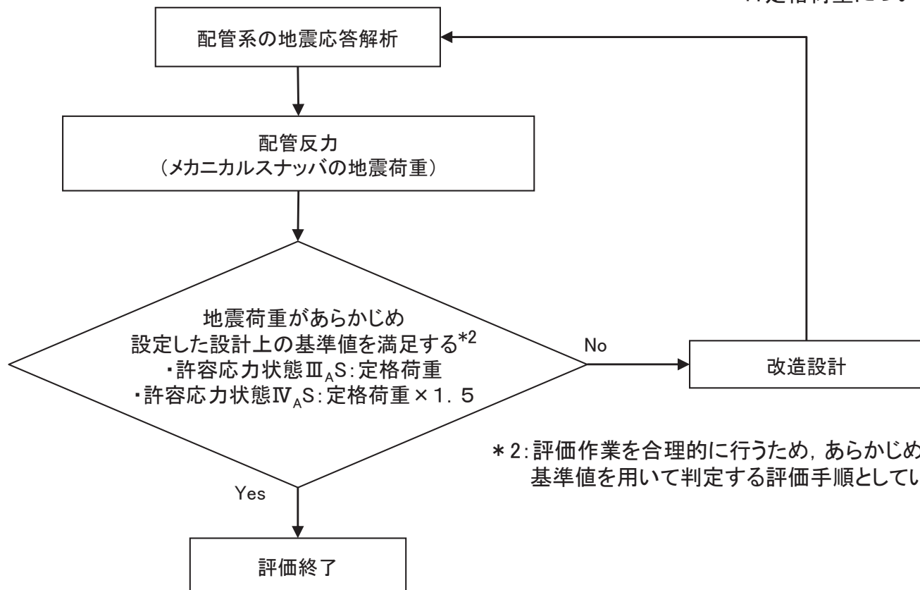
図2 既工認における評価手順
