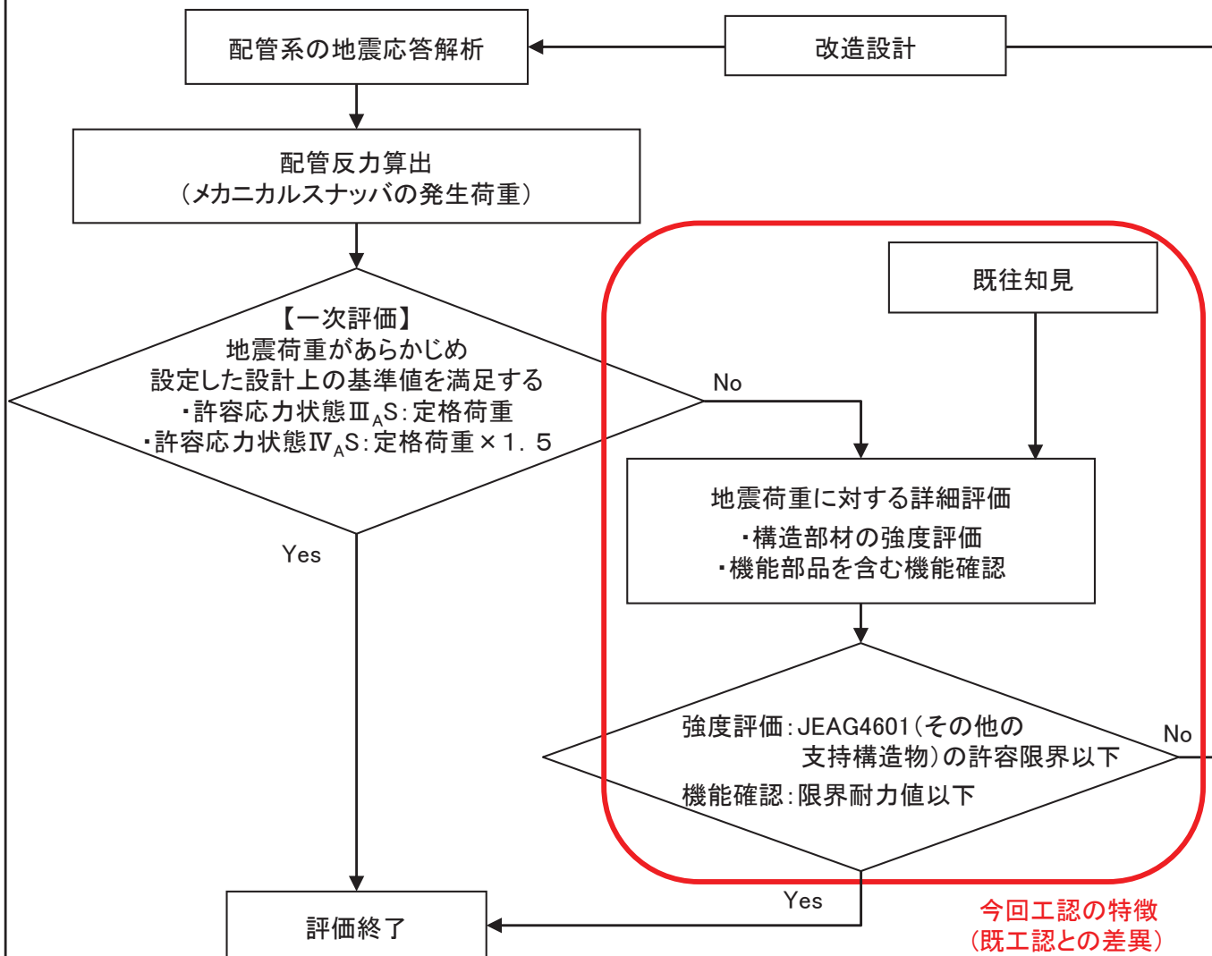
図3 今回工認における評価手順
