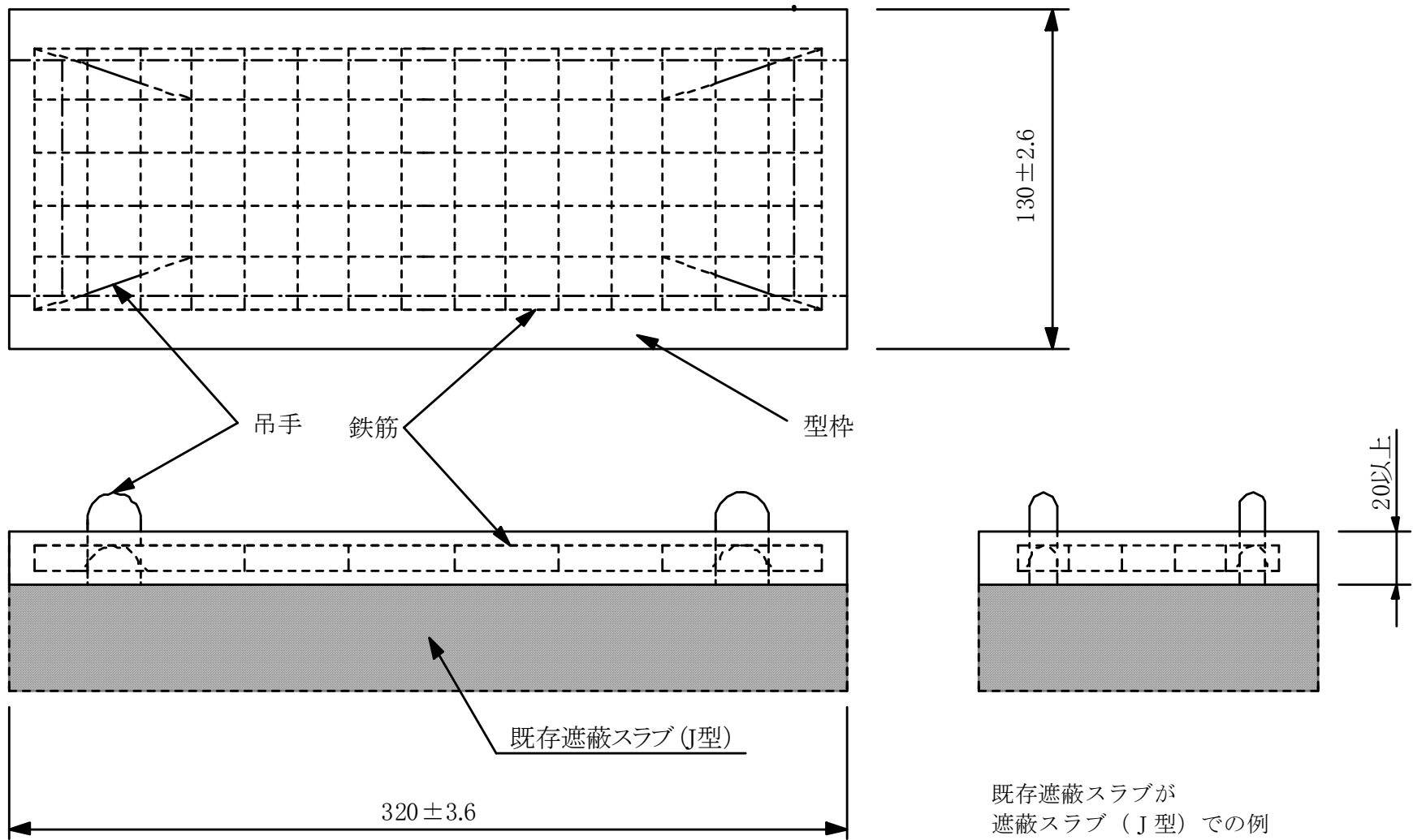
別図 打ち増しの構造
