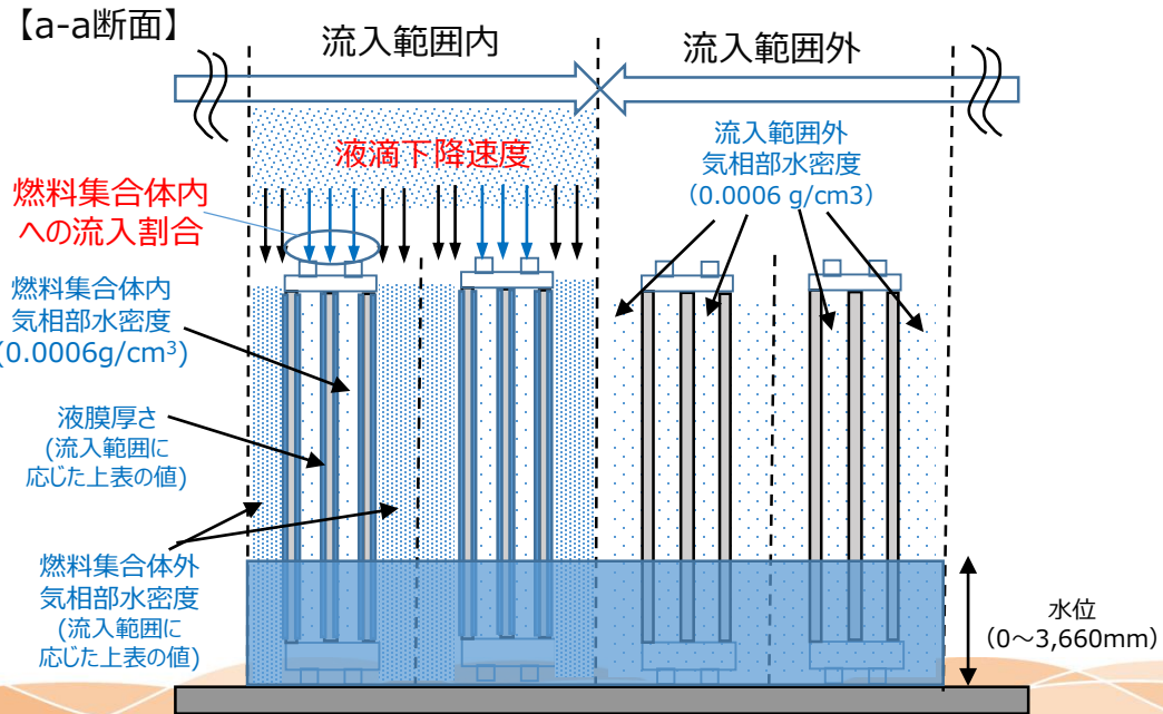
図 臨界計算コードへの入力となる水分条件 概要
