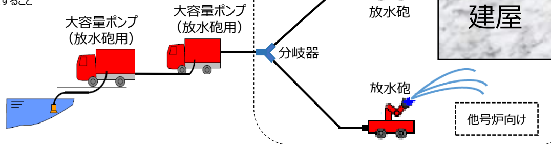
図 整備している手順に基づく系統構成（放水砲による放水手順）
