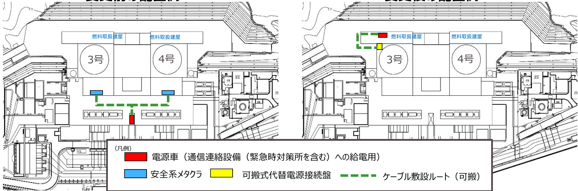
変更前の配置例
