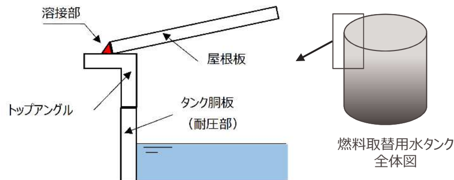
【燃料取替用水タンク（屋根板概要図）】
