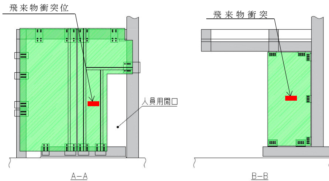
第 5 - 9 図 二辺支持防護板 飛来物衝突評価位置②
