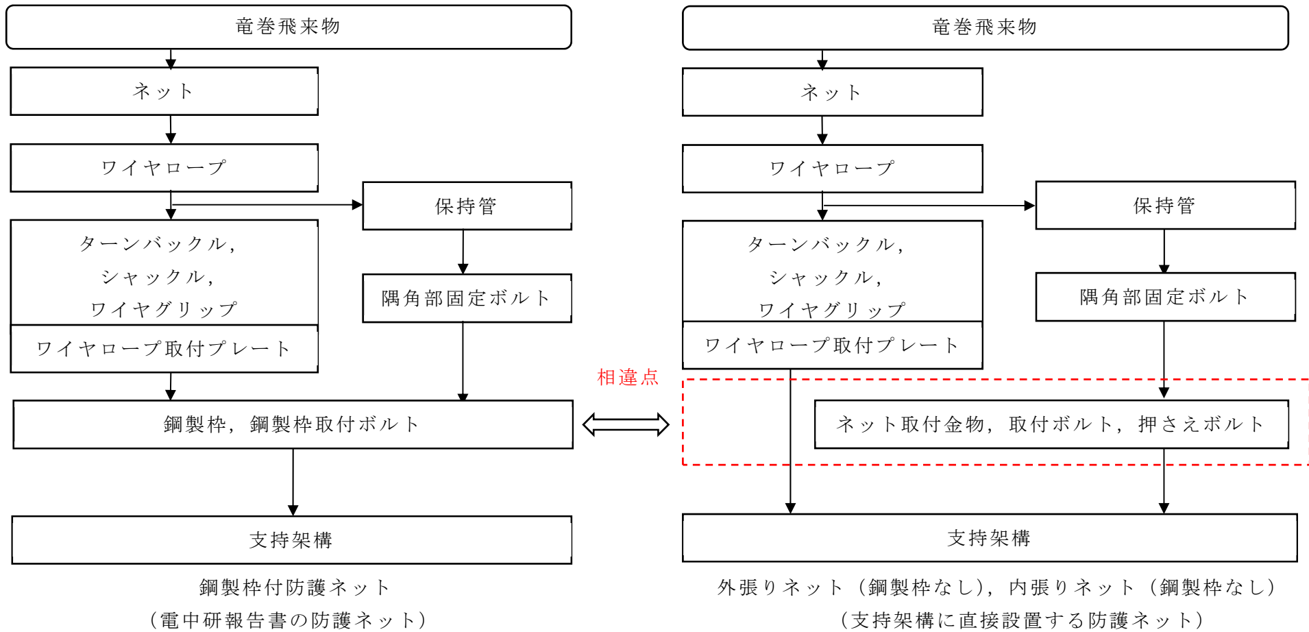
第5-5図 防護ネットの荷重伝達機構の比較
