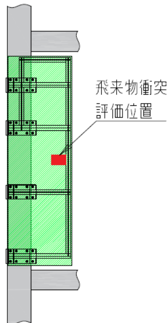
第 5-7 図 一辺支持防護板 飛来物衝突評価位置
