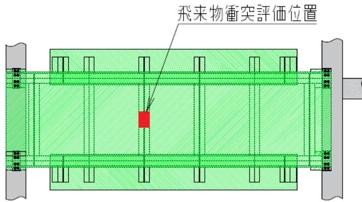
第 5 - 8 図 二辺支持防護板 飛来物衝突評価位置
