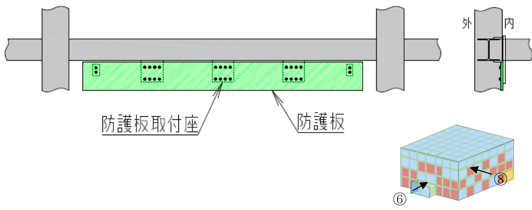
第 3-13 図 ⑦防護板
