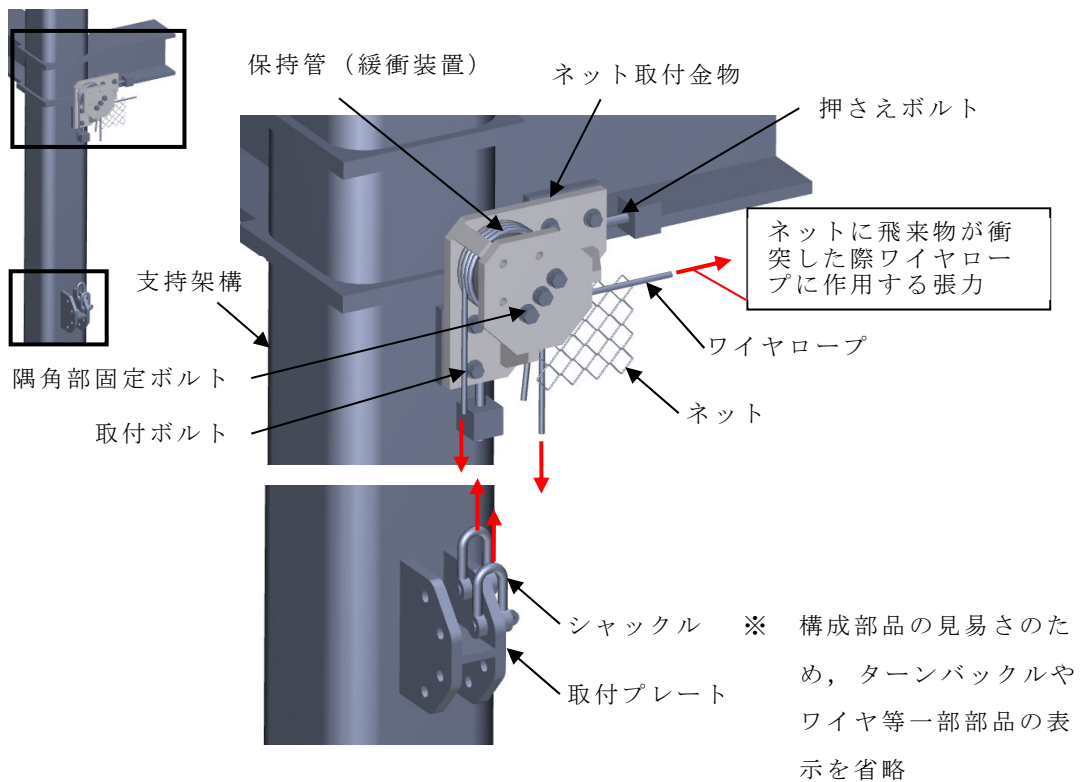
第3-5図 外張りネット（鋼製枠なし） 支持架構への取付部拡大図
