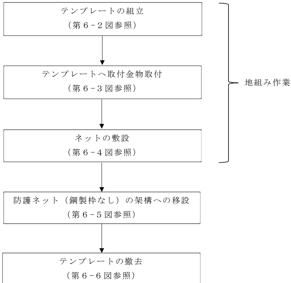
第6-1図 防護ネット（鋼製枠なし）の組立フロー
