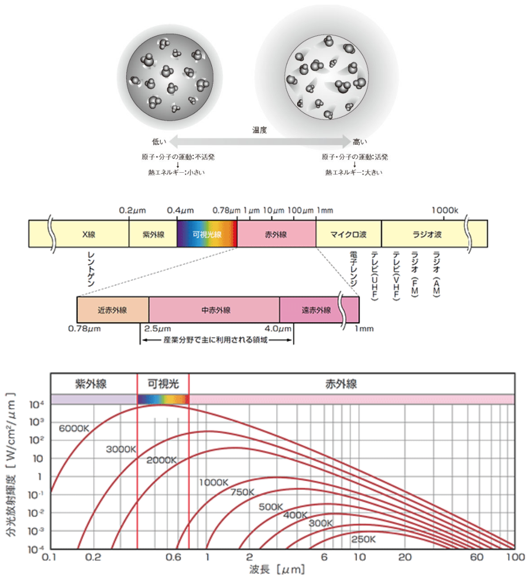
第4-6図 温度測定の実理
