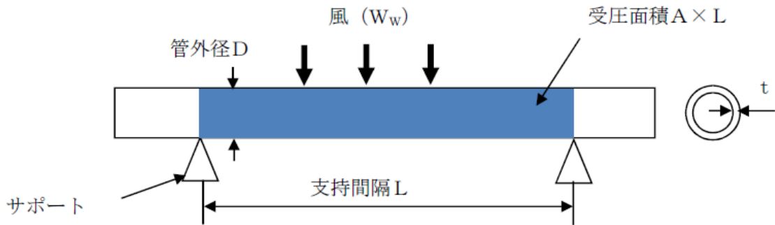
第 4-5 図 配管モデル図
