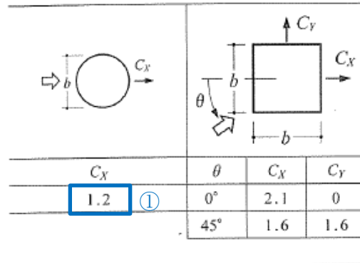
第4-4図 部材の風力係数
