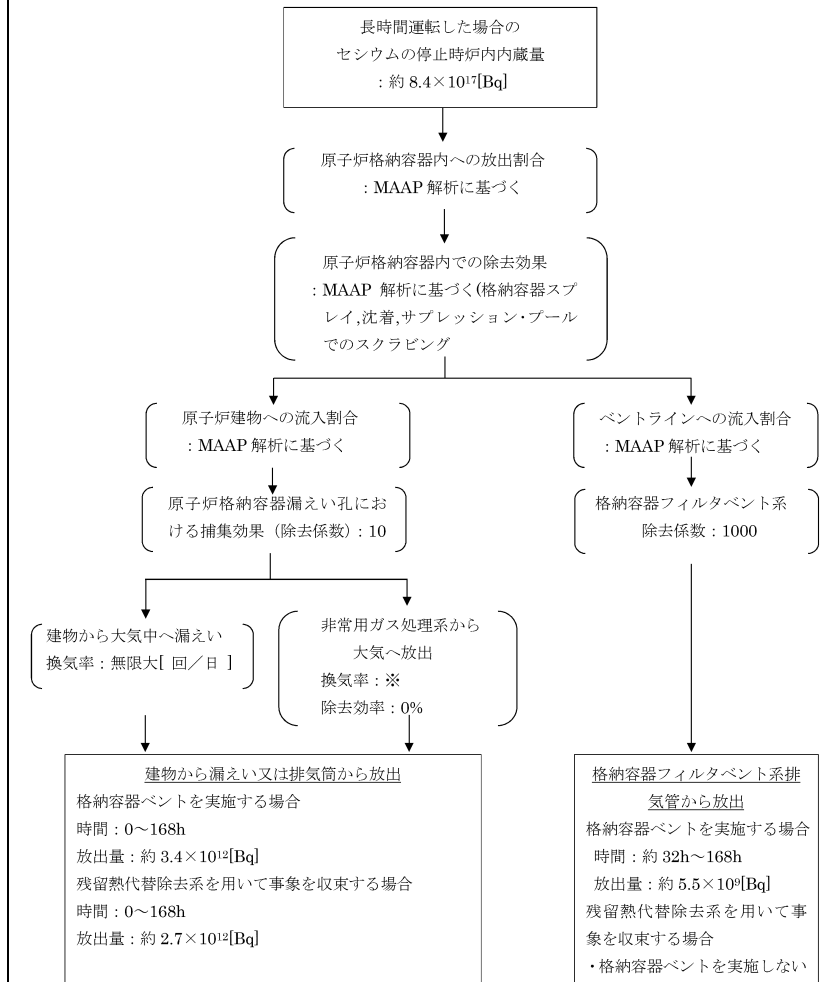
図3 セシウムの大気放出過程
