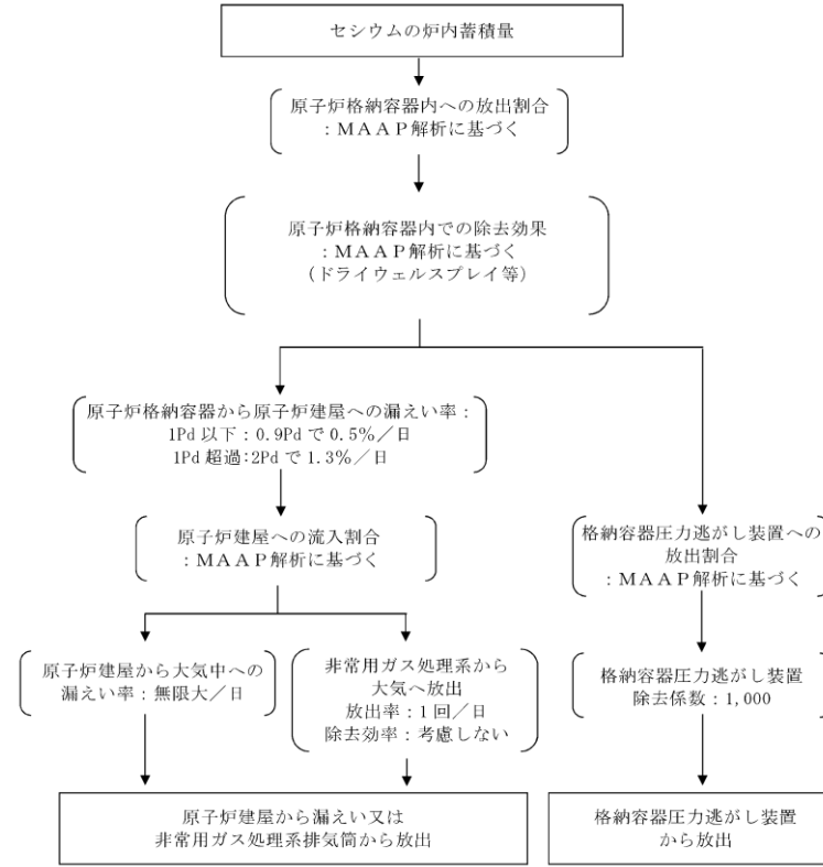
第3図 セシウムの大気放出過程
