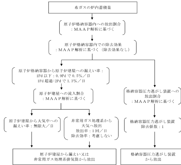
第1図 希ガスの大気放出過程
