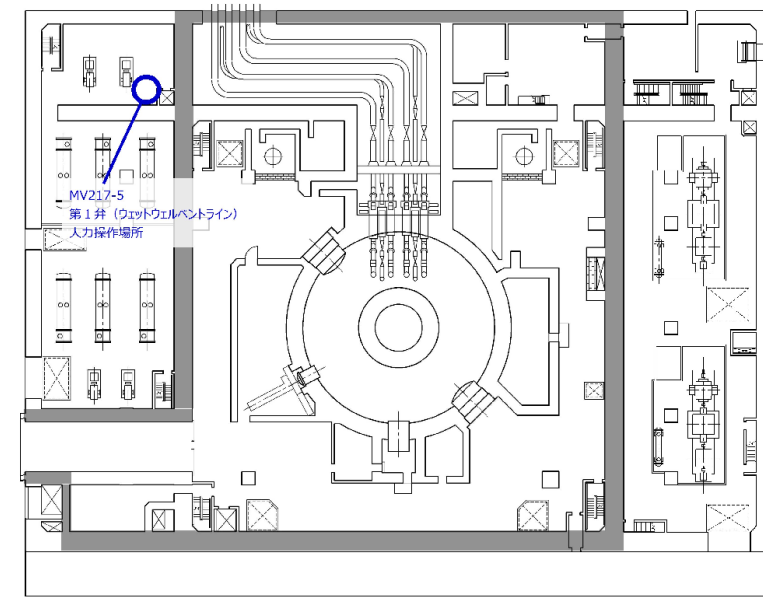
第8図 第1弁（W/Wベント）操作場所（原子炉建物地上1階）
