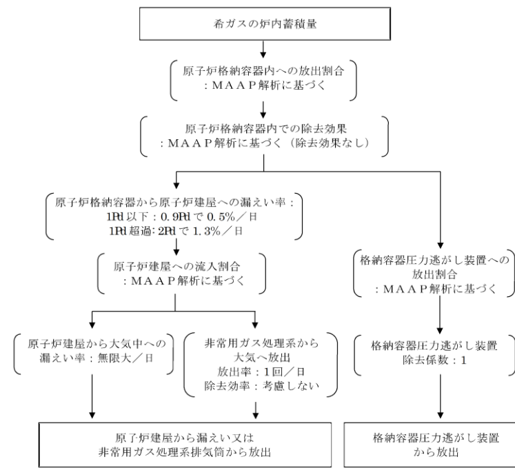
第21図 希ガスの大気放出過程
