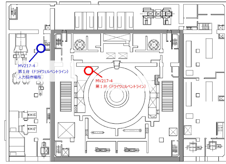
R/B 2FL (EL23800)
