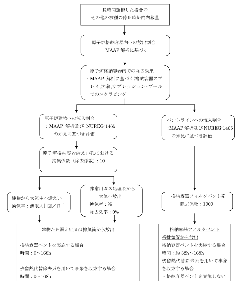
図4 其他核種の大気放出過程
