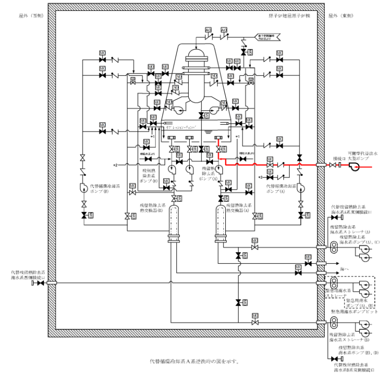
第5図 残熱除去系吸入ストレーナ逆洗操作の系統構成について
