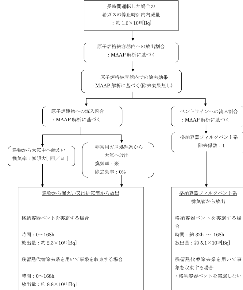
図1 希ガスの大気放出過程
