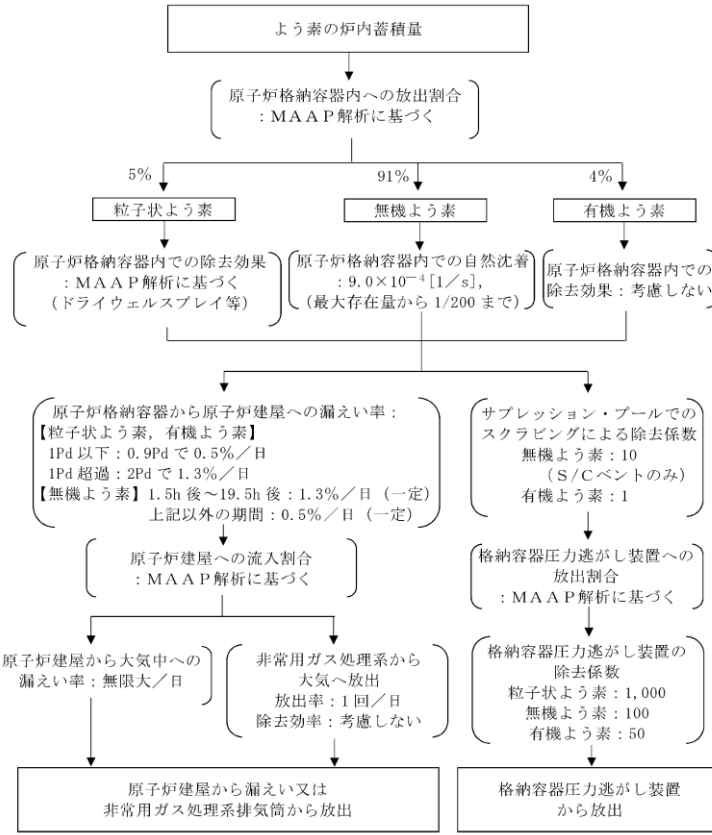
第2図 よう素の大気放出過程
