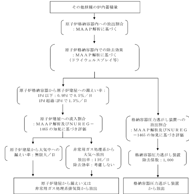
第4図 其他核種の大気放出過程
