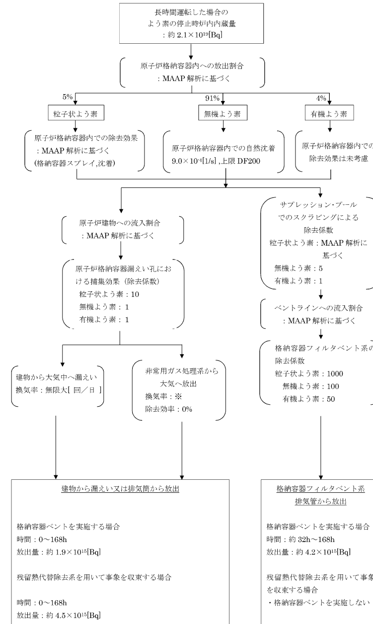
図2 よう素の大気放出過程
